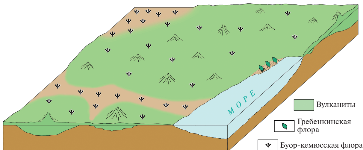
Рис. 7. Схема распространения флоры гребенкинского и буор-кемюсского типов в разных ландшафтных обстановках на Северо-Востоке Азии в позднем альбе–раннем туроне (по Щепетов и др., 2019, с изменениями).
