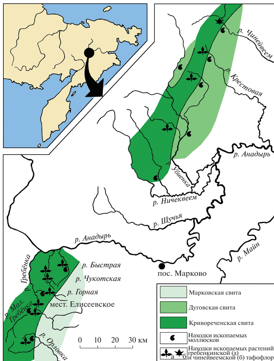
Рис. 2. Распространение флороносных отложений кривореченской свиты и перекрывающих образований дуговской и марковской свит в среднем течении р. Анадырь и приуроченные к ним местонахождения ископаемых моллюсков и растений гребенкинской и чинейвеевской тауфлор (по Герман, 2011, с изменениями).
