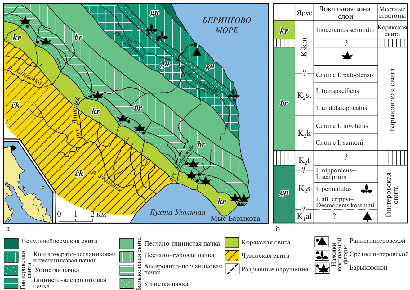
Рис. 4. Схематическая геологическая карта отложений северного побережья бухты Угольной (а) и выделяемые здесь стратоны (б) (по Пергамент, 1966, с изменениями).
