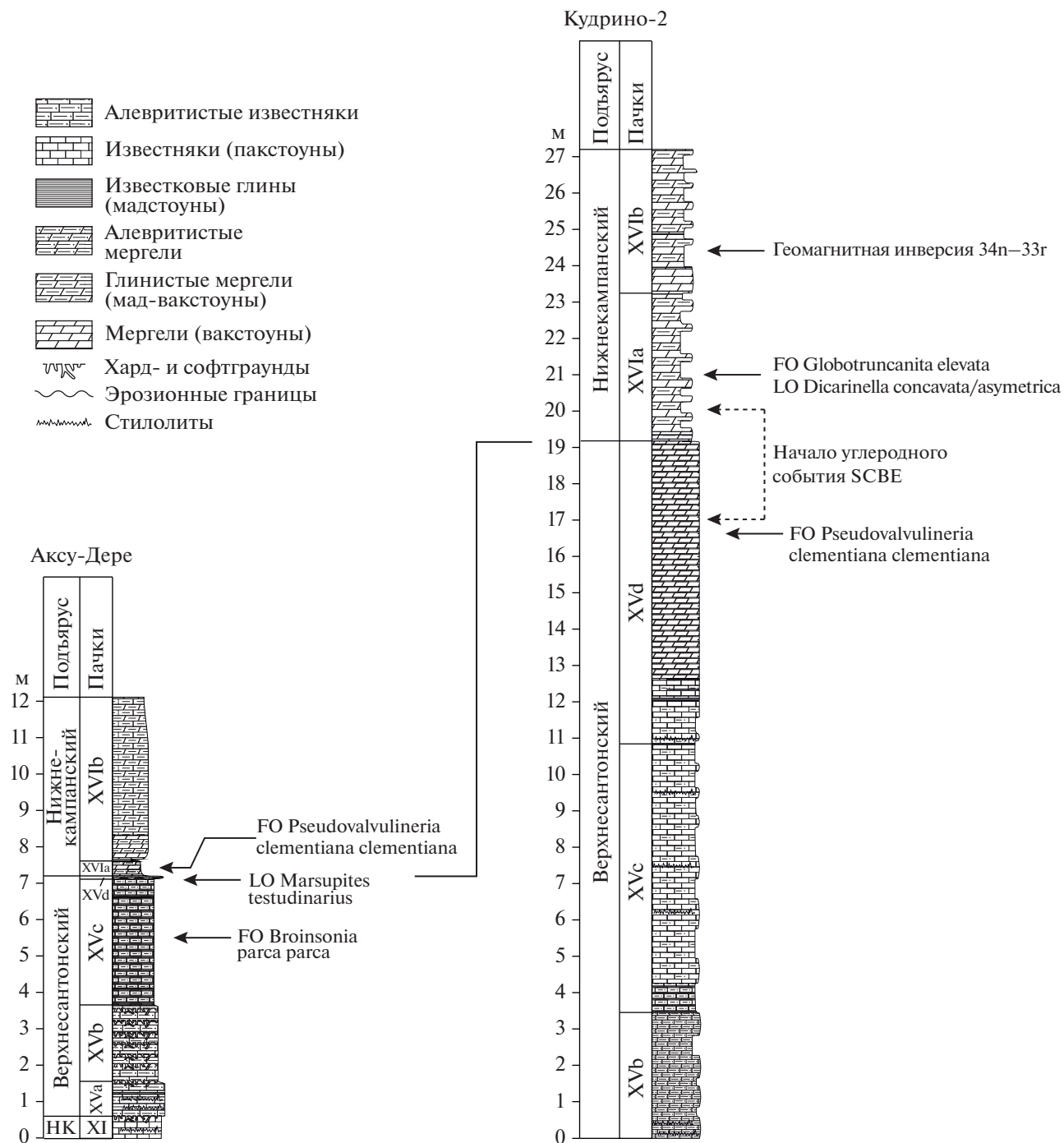
Рис. 12. Последовательность событий в пограничном интервале сантона–кампана разрезов Кудрино-2 и Аксу-Дере.
