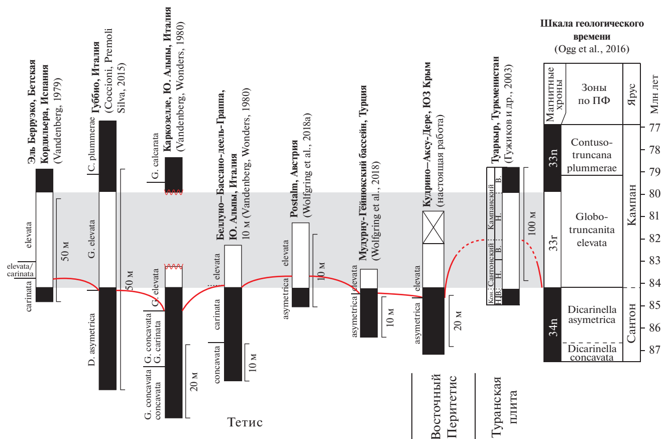
Рис. 10. Результаты палеомагнитной калибровки биостратиграфических границ, обоснованных по планктонным фораминиферам.
