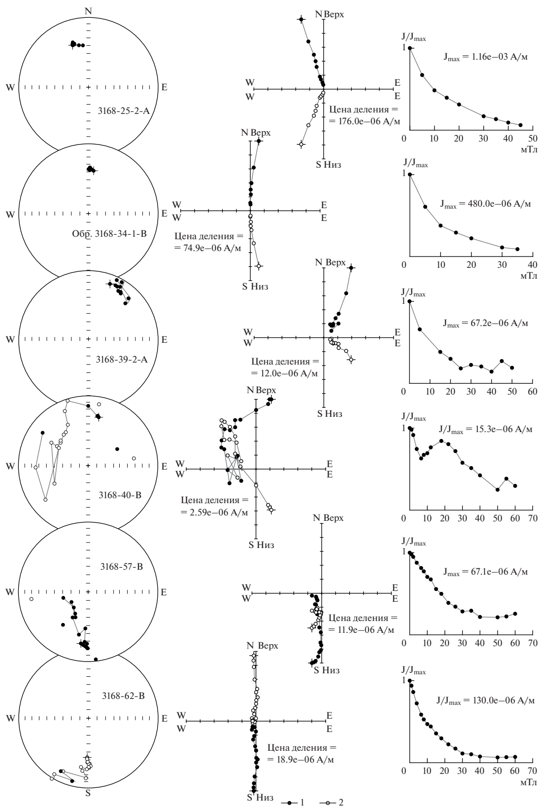
Рис. 3. Результаты компонентного анализа (слева направо): изображения на полярных стереопроециях изменений векторов J_n в процессе магнитных чисток (в стратиграфической системе координат); диаграммы Зийдервельда (в стратиграфической системе координат); графики размагничивания образцов.
