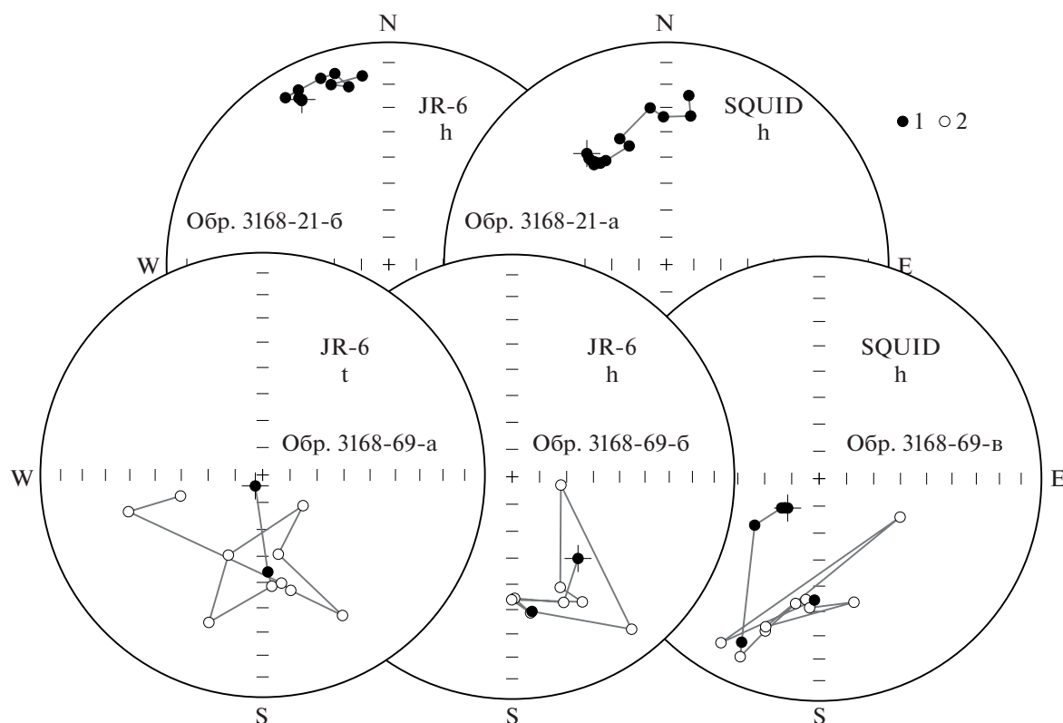
Рис. 2. Сопоставление результатов магнитных чисток (h — переменным полем, t — температурой) на спин-магнитометре JR-6 в лаборатории петрофизики СГУ (Саратов) и на криогенном магнитометре 2G-Enterprises (SQUID) в ИФЗ РАН (Москва). Полярные стереопроекции приведены в стратиграфической системе координат. Условные обозначения: 1, 2 — проекции J_n на нижнюю (1) и верхнюю (2) полусферы.
