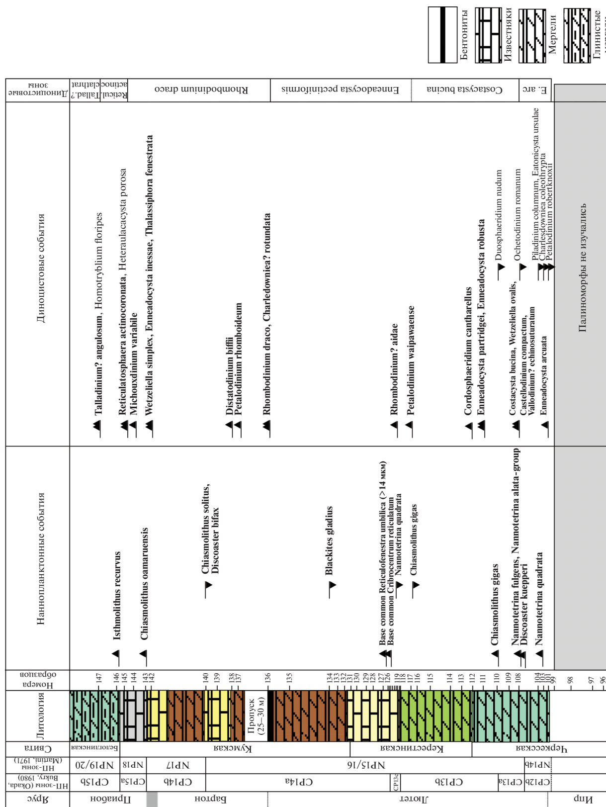
Рис. 3. Калибровка диноцистовых событий (датумов) и диноцистовых зон с датумами и зонами по наннопланктону в разрезе Хей. НП-зоны — зоны по наннопланктону, Reticul. actinos — Reticulatosphaera actinocoronata, Tallad.? clathrat — Talladinium? clathrat; полужирным шрифтом выделены наиболее важные виды.
