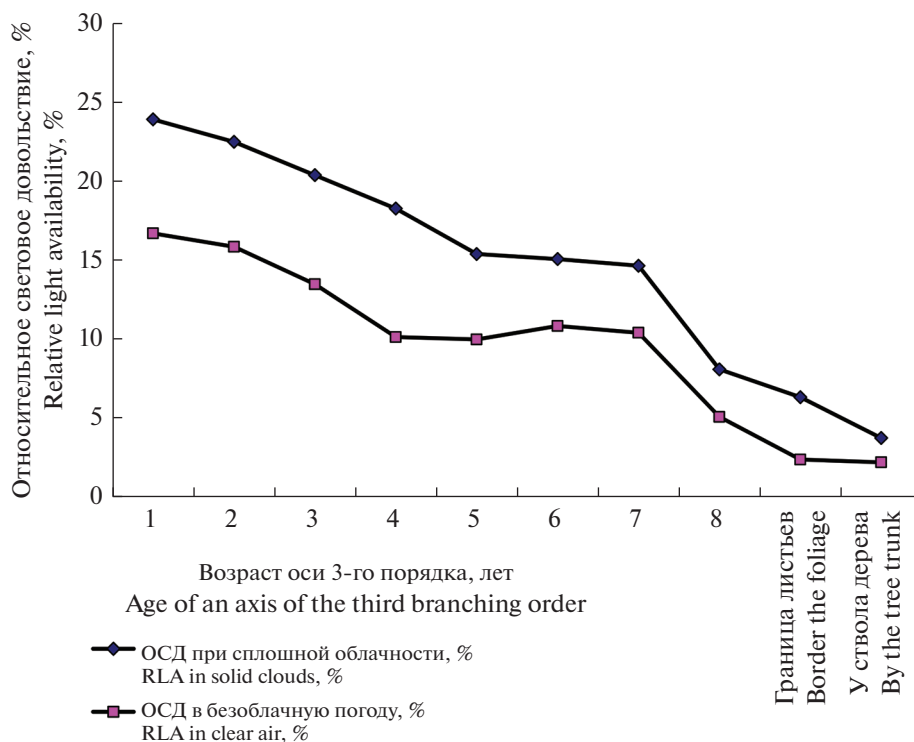
Рис. 1. Величина относительного светового довольствия на различной глубине кроны Pseudotsuga menziesii в безоблачную погоду и при сплошной облачности.
