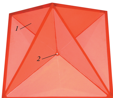
Рис. 4. Внешний вид РОО кругового действия со светоотражающими гранями. 1 – светоотражающая пленка, 2 – светоизлучающий диод.
