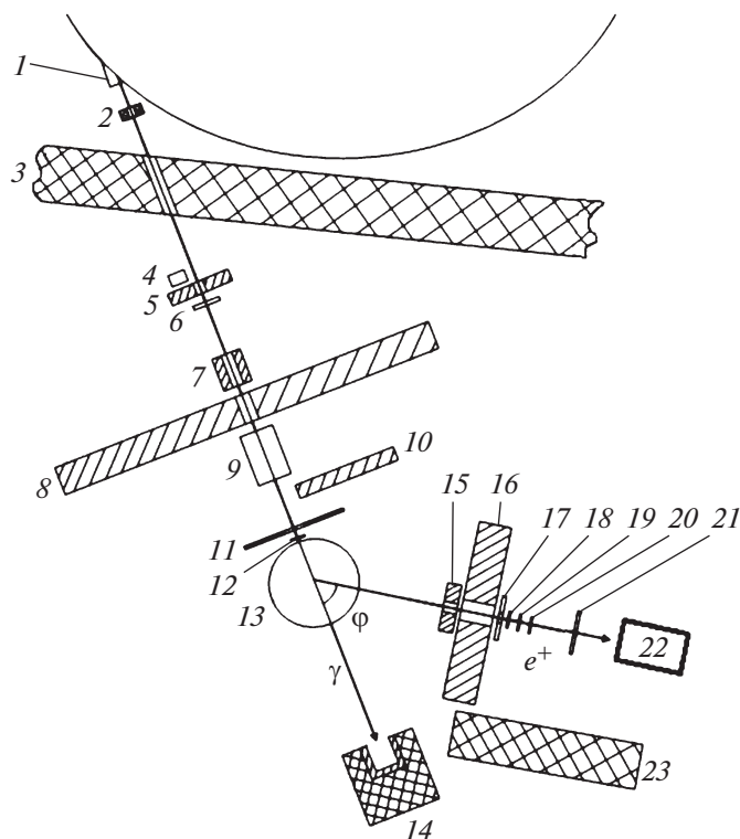
Рис. 2. Схема калибровочного квазимонохроматического пучка вторичных электронов. 1 — выходное окно камеры ускорителя; 2 — коллиматор; 3 — бетонная стена ускорительного зала; 4 — монитор “растяжки”; 5, 7, 16 — коллиматоры; 6 — монитор пучка; 8 — протяженная свинцовая стенка; 9 — очищающий магнит СП-3; 10 — дополнительная свинцовая стенка; 11 — металлическая плита; 12 — конвертер; 13 — магнит СП-57; 14 — поглотитель фотонного пучка; 15 — дополнительный коллиматор перед основным; 17 — сцинтилляционный счетчик антисовпадений; 18–21 — сцинтилляционные счетчики; 22 — калибруемый детектор; 23 — бетонный блок.
