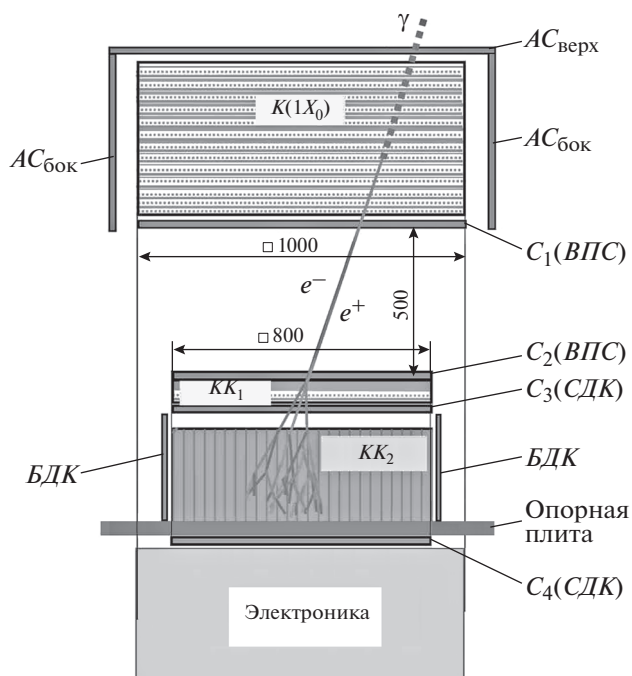
Рис. 3. Схема \gamma -телескопа ГАММА-400. АС – система антисовпадений (верхний АС верх и боковые АС бок детекторы); К – конвертер-трекер; C 1 , C 2 – сцинтилляционные детекторы времяпролетной системы (ВПС); C 3 , C 4 – сцинтилляционные детекторы калориметра (СДК); KK 1 – позиционно-чувствительный калориметр; KK 2 – электромагнитный калориметр; БДК – боковые детекторы (4 шт.) калориметра KK 2 .
