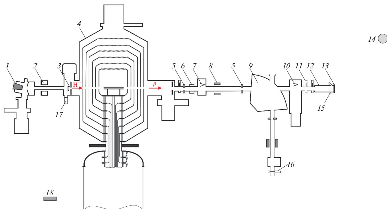
Рис. 1. Схема экспериментальной установки. 1 — источник отрицательных ионов водорода; 2 — магнитная линза; 3 — входная охлаждаемая диафрагма ускорителя; 4 — ускоритель-тандем с вакуумной изоляцией; 5 — охлаждаемая диафрагма с апертурой 26 мм; 6 — бесконтактный датчик тока; 7 — выдвижной цилиндр Фарадея в диагностическом баке на выходе из ускорителя; 8 — корректор; 9 — поворотный магнит; 10 — выдвижной цилиндр Фарадея в диагностическом баке за поворотным магнитом; 11, 16 — шиберы; 12 — вакуумная камера; 13 — литевая мишень; 14 — дозиметр нейтронов; 15 — патрубки с окнами для наблюдения; 17 — проволочный сканер; 18 — детектор нейтронов.
