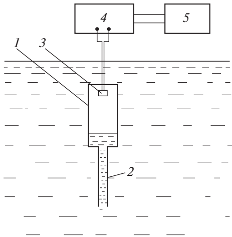
Рис. 1. Схема гидрофона. 1 – резервуар; 2 – труба; 3 – пирозлемент; 4 – усилитель; 5 – регистрирующее устройство.
