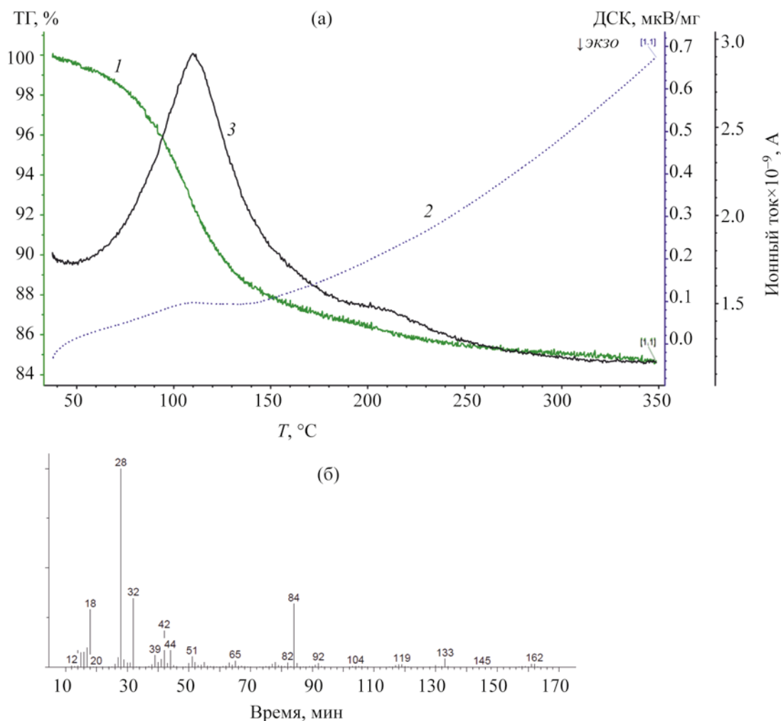
Рис. 6. Данные ТГ (а) и масс-спектрометрии (б) образца № 2 без глицерина. 1 – ТГ, 2 – ДСК, 3 – ТГС.
