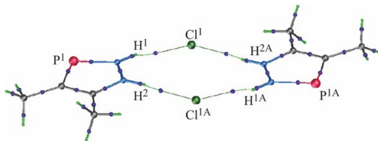
Рис. 5. Экспериментально-теоретический молекулярный граф, визуализирующий \text{H}\cdots\text{Cl} взаимодействия между соседними стопками молекул 7 . Приведены только критические точки (3, –1). Индексом «А» отмечена молекула из соседней стопки.
