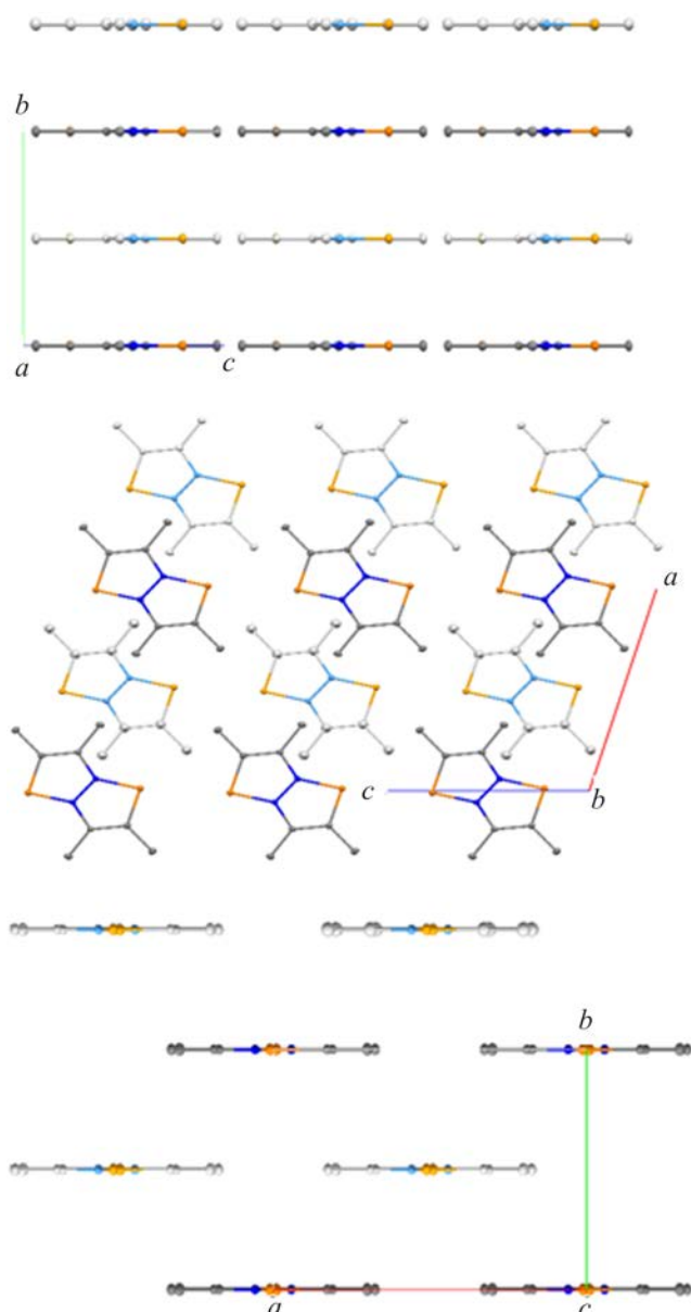
Рис. 7. Фрагмент кристаллической упаковки соединения 8 в трех проекциях. Атомы водорода не приведены для ясности. Молекулы нечетных и четных слоев приведены в светлом и темном оттенках соответственно.
