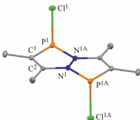
Рис. 1. Общий вид молекулы соединения 4 в кристалле. Тепловые эллипсоиды приведены с 50%-ной вероятностью. Атомы водорода опущены для ясности. Операция симметрии, используемая для генерации эквивалентных атомов в комплексе 4 (A): -x+1, -y+1, -z+1 . Избранные длины связей (Å) и углы (град): P 1 –N 1A 1.6939(10), P 1 –C 1 1.7971(12), P 1 –Cl 1 2.1837(4), N 1 –N 1A 1.4055(17), N 1 –C 2 1.3946(14), C 1 –C 2 1.3526(15); C 1 P 1 N 1A 88.19(5), C 1 P 1 Cl 1 98.70(4), N 1A P 1 Cl 1 104.29(4), N 1A N 1 P 1A 114.73(9), C 2 N 1 P 1A 133.70(7), C 2 N 1 N 1A 110.01(11).
