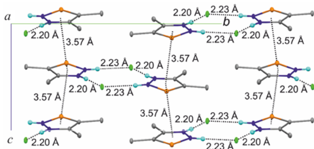
Рис. 3. Фрагмент кристаллической упаковки соединения 7 . Атомы водорода, не принимающие участие в межмолекулярных \text{NH}\cdots\text{Cl} взаимодействиях, не приведены для ясности.
