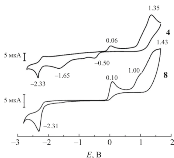
Рис. 8. Циклическая вольтамперометрия соединений 4 и 8 в ДМФА, \nu 100 мВ/с (5мМ., электролит 0.1 М. ТВАРФ 6 , потенциалы приведены относительно Ag/AgCl).
