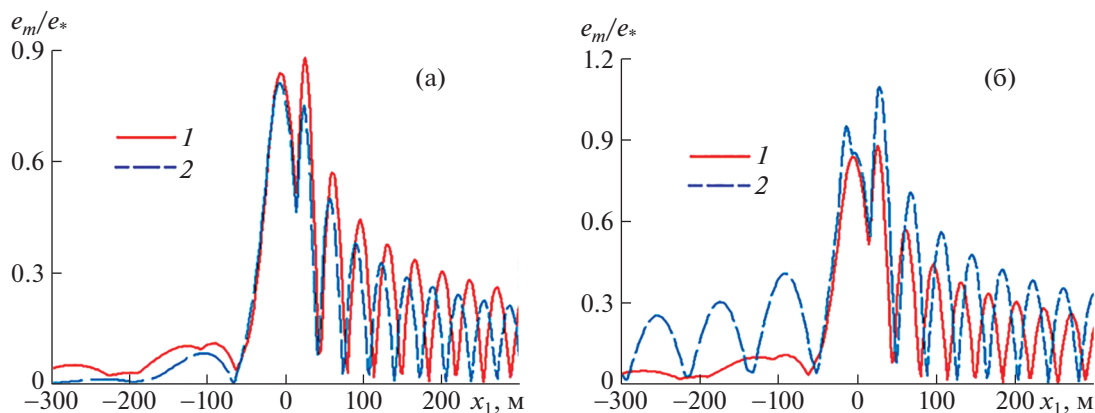
Рис. 3. Зависимости от координаты x_1 максимальных деформаций ледяного покрова e_m/e_* при y_1 = 0 , \bar{Q} = 0 , V = 20 м/с: (а–б) – \psi = 0, \pi ; 1–2 – S = 0, 0.4 .
