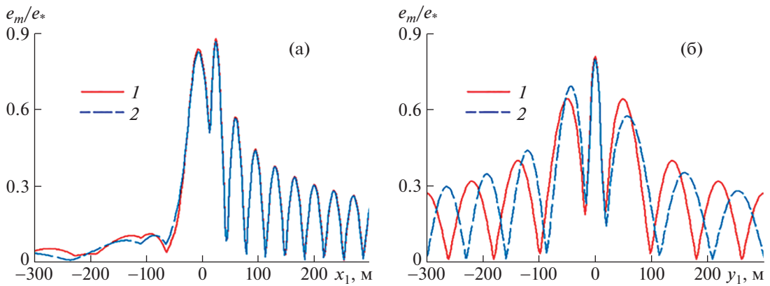
Рис. 5. Зависимости от координаты x_1 при y_1 = 0 (а) и от координаты y_1 при x_1 = 0 (б) максимальных деформаций ледяного покрова e_m/e_* при \bar{Q} = 0 , V = 20 м/с, \psi = \pi/2 : 1–2 – S = 0, 0.4 .
