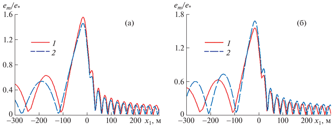
Рис. 4. Зависимости от координаты x_1 максимальных деформаций ледяного покрова e_m/e_* при y_1 = 0 , \bar{Q} = 1.5 , V = 20 м/с: (а–б) – \psi = 0, \pi ; 1–2 – S = 0, 0.4 .
