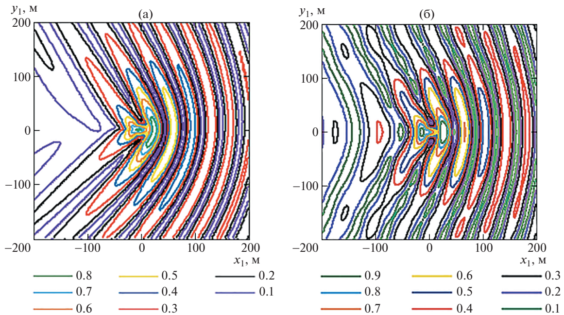
Рис. 6. Изолинии максимальных деформаций ледяного покрова e_m/e_* при \bar{Q} = 0 , V = 20 м/с, S = 0.4 : (а–б) – \psi = \pi/2, \pi .
