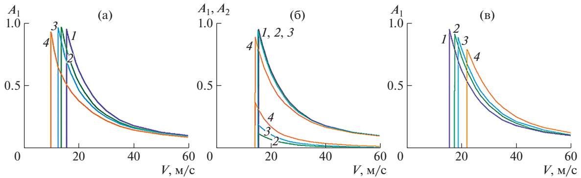
Рис. 1. Зависимости безразмерных коэффициентов волновых сил A_1 , A_2 от скорости движения нагрузки при \bar{Q} = 0 : (а–в) – \psi = 0, \pi/2, \pi ; 1–4 – S = 0, 0.3, 0.5, 1 .
