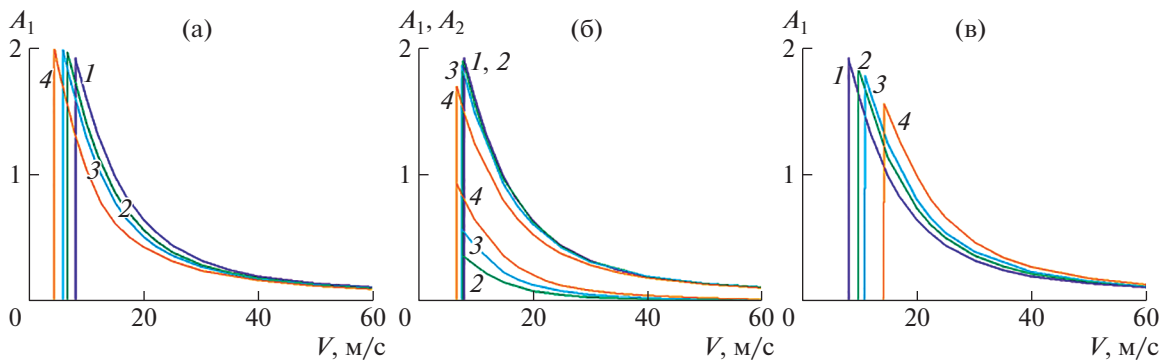
Рис. 2. Зависимости безразмерных коэффициентов волновых сил A_1 , A_2 от скорости движения нагрузки при \bar{Q} = 1.5 : (а–в) – \psi = 0, \pi/2, \pi ; 1–4 – S = 0, 0.3, 0.5, 1 .
