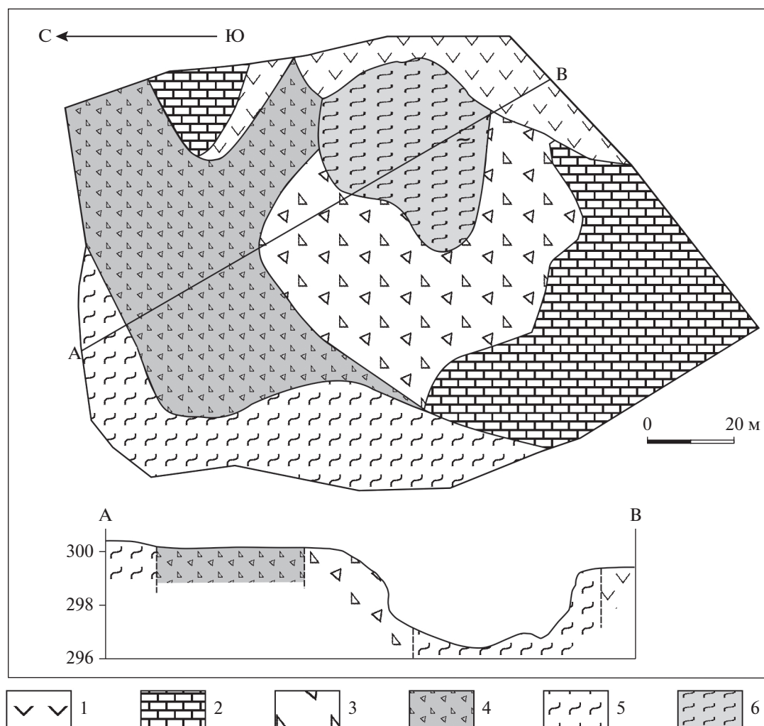
Рис. 3. Зарисовка полотна полигона россыпной золотодобычи, руч. Глухариный, р.л. 113–115 (А) и профиль полотна полигона по линии АВ (В).
