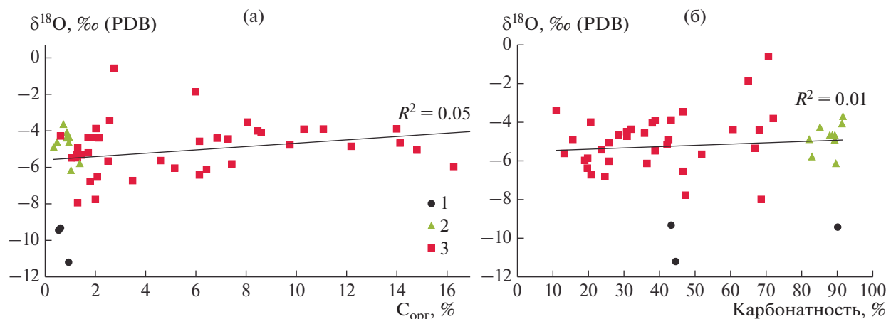
Рис. 5. Корреляционные диаграммы \delta^{18}\text{O} — C_{\text{орг}} (а) и \delta^{18}\text{O} —карбонатность (б) для пород верхнефаменского сланценового разреза Припятского прогиба (Любанское месторождение горючих сланцев, скв. 168). 1 — породы с явными постдиагенетическими изменениями, 2 — известняки и глинистые известняки, 3 — мергели, глинистые мергели и карбонатсодержащие глины; R^2 — коэффициент регрессии.
