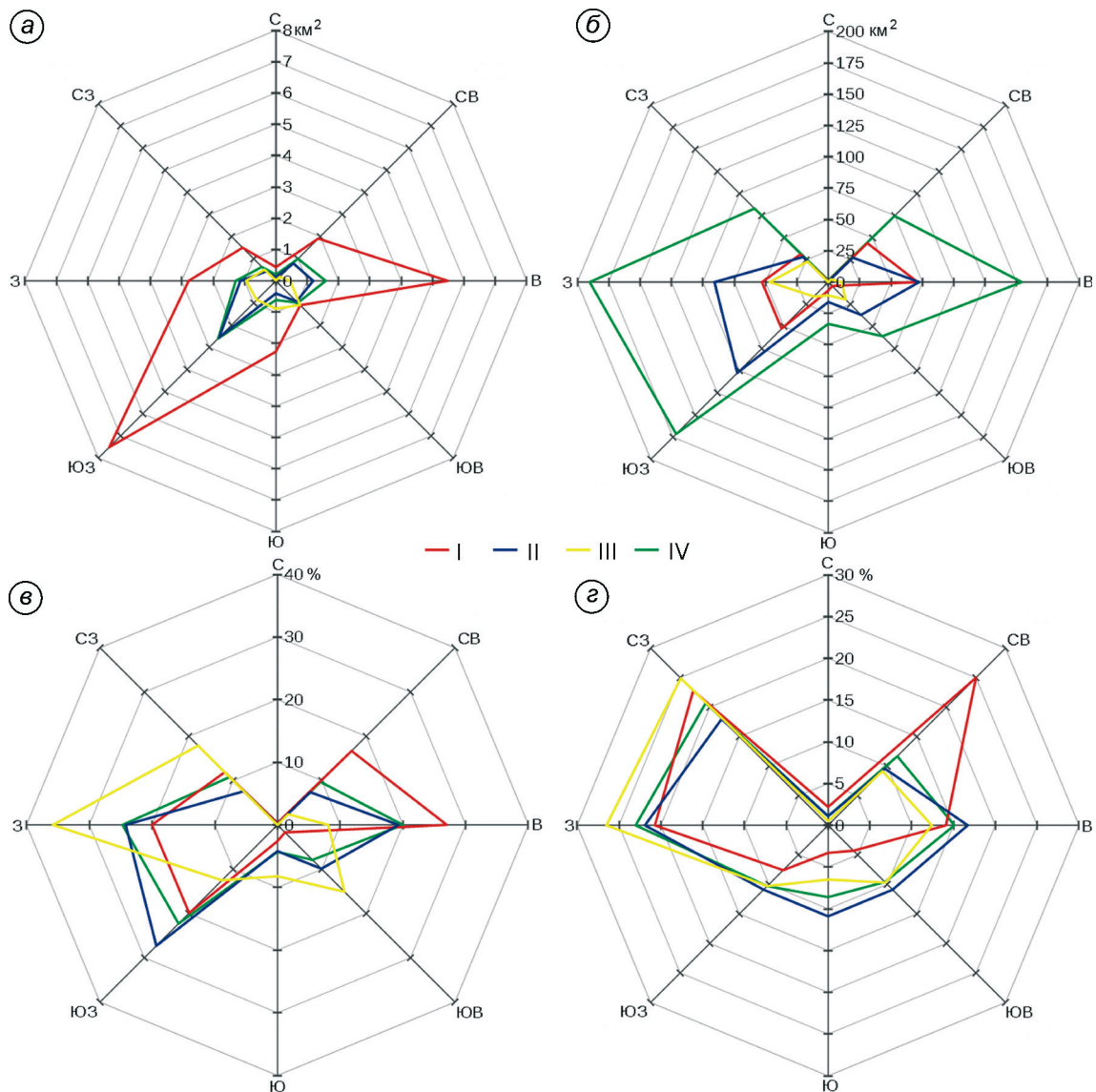
Рис. 2. Изменение ряда характеристик оледенения Камчатки в районах с разным типом зависимости ледников от экспозиции:
