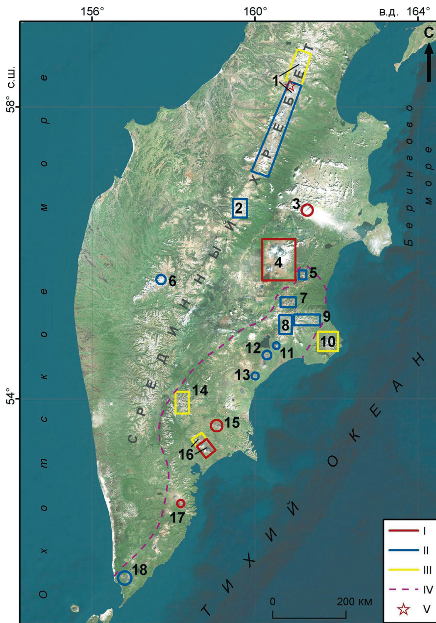
Рис. 1. Районы оледенения Камчатки:
