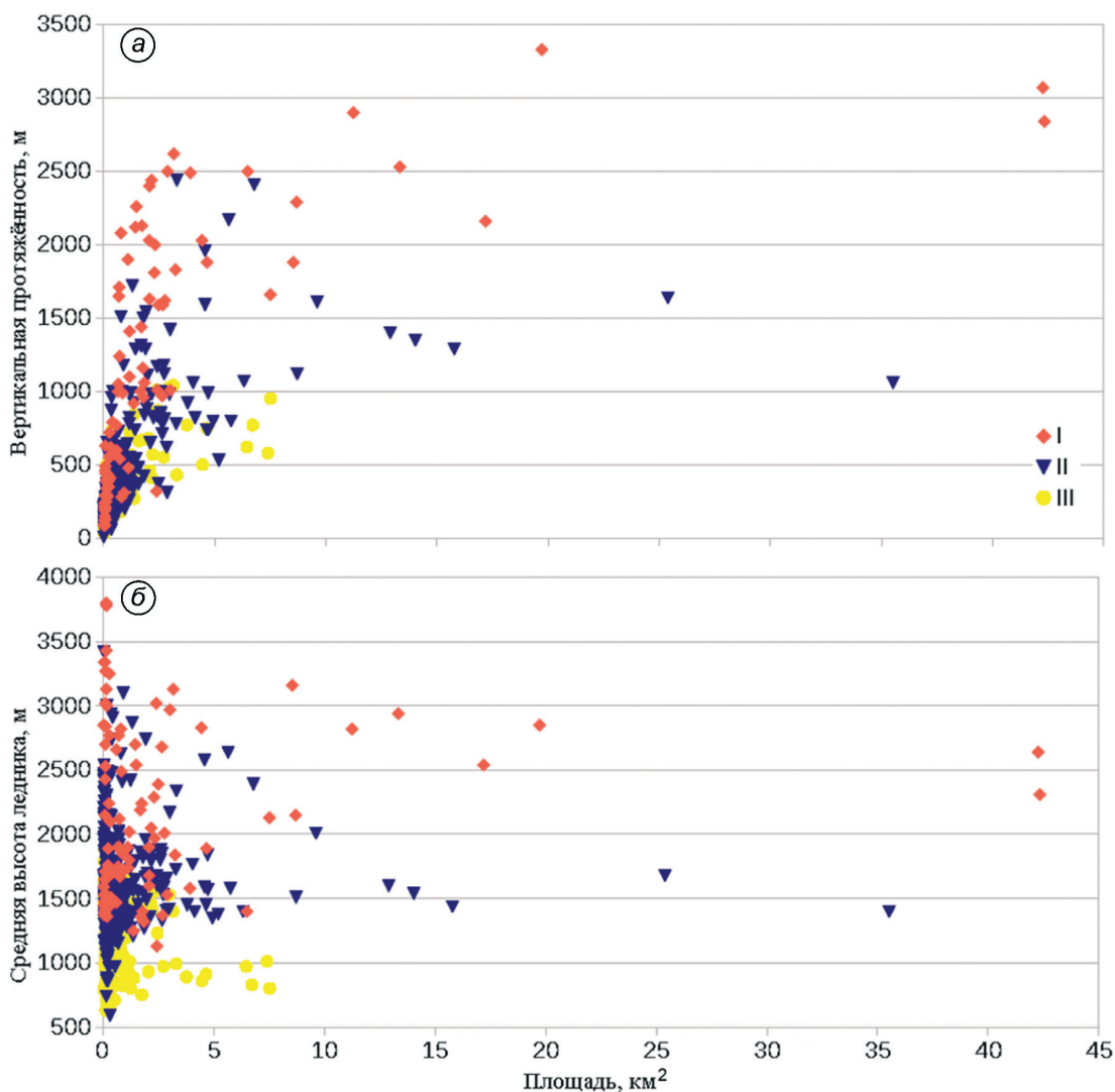
Рис. 3. Вертикальная протяжённость ледников Камчатки (а) и средние высоты ледников (б) разной площади в трёх типах районов оледенения Камчатки.
