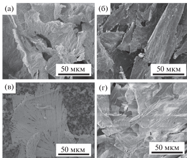
Рис. 7. Микрофотографии СЭМ гибридных систем: (а) \text{ОГ}/\text{ZnPc}_{16} ; (б) \text{ОГ}/\text{Zn}(\text{OAc})_2/\text{ZnPc}_{16} , высушенного под вакуумом и (в) высушенного с помощью лиофильной сушки; (г) контроль — \text{ОГ}/\text{Zn}(\text{OAc})_2 .
