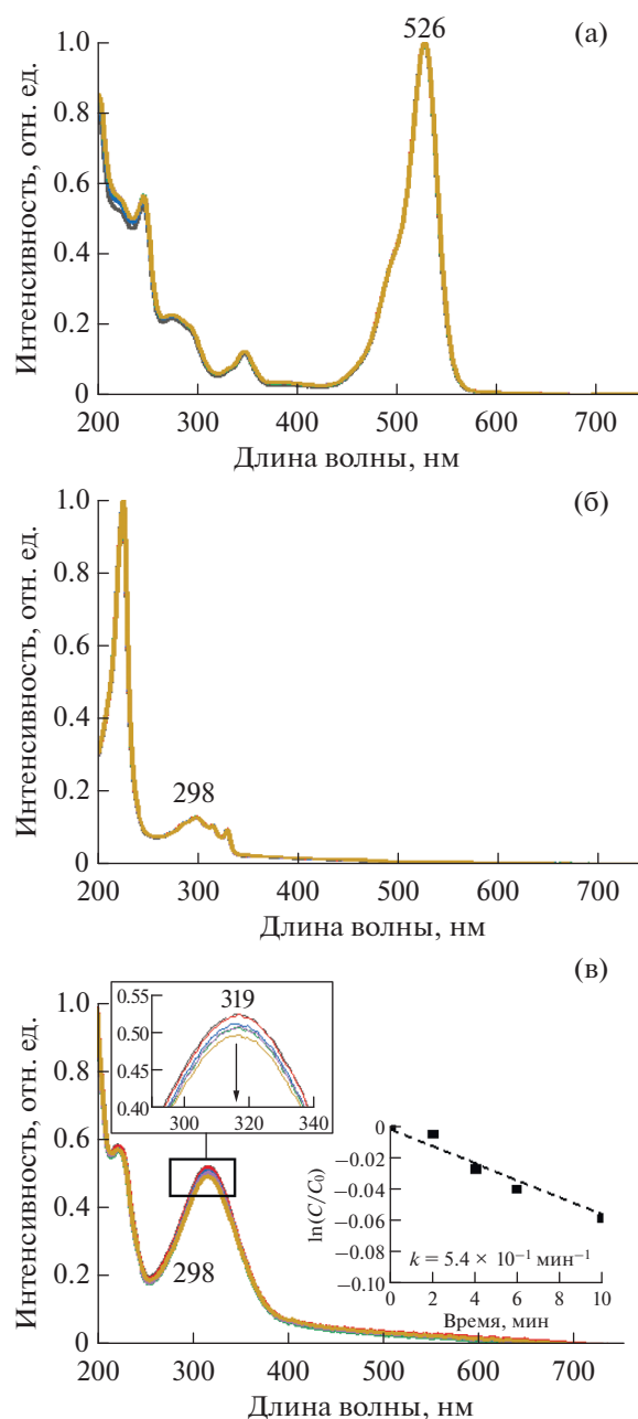
Рис. 12. Электронные спектры поглощения и соответствующие кинетические зависимости фотодеградации для растворов (а) Rh6G, (б) ДГН и (в) НФ в присутствии ОГ/ \text{ZnPc}_{16} при облучении фитолампой в течение 10 минут, снятые с интервалом 2 мин. Вставка: увеличенное изображение спектров поглощения НФ в области 280–340 нм.
