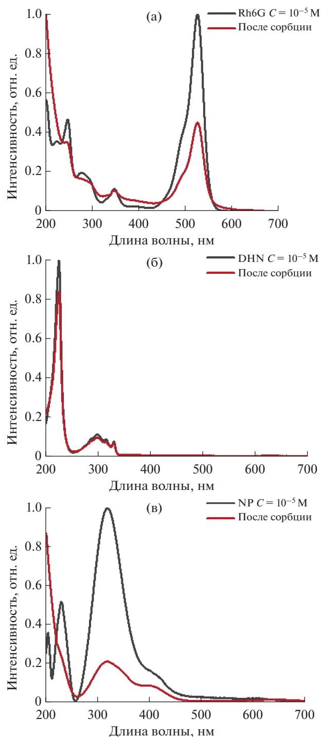
Рис. 11. Электронные спектры поглощения растворов (а) Rh6G, (б) ДГН и (в) НФ, после адсорбции и достижения равновесия в присутствии ОГ/ \text{Zn}(\text{OAc})_2/\text{ZnPc}_{16} .
