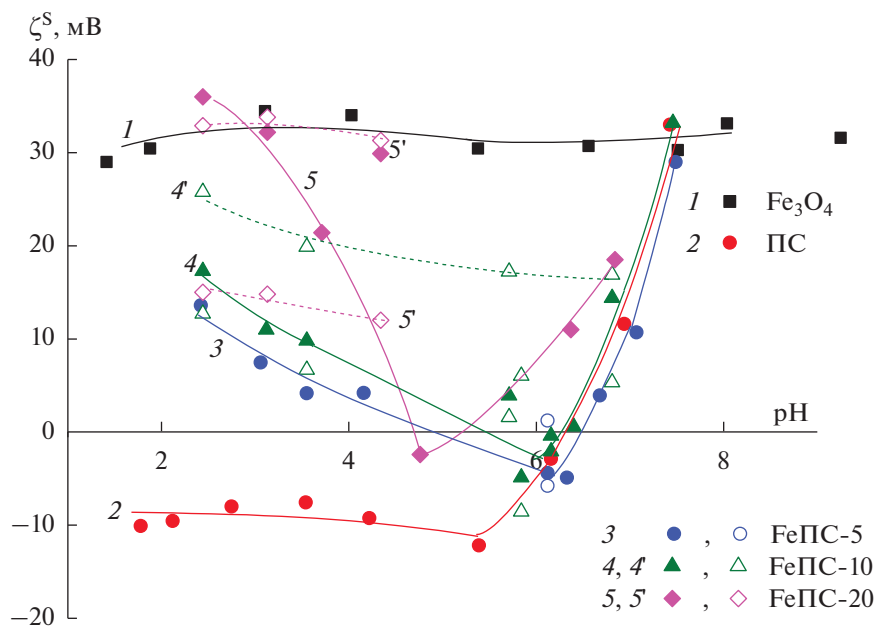
Рис. 9. Зависимость электрокинетического потенциала частиц исследованных образцов от pH при ионной силе 10^{-2} М раствора \text{NiCl}_2 (закрашенные точки – средние значения дзета-потенциала, незакрашенные точки – значения пиков на кривой распределения дзета-потенциала).
