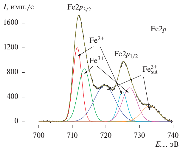
Рис. 3. Спектр РФЭС 2p-электронов железа в порошке магнетита.
