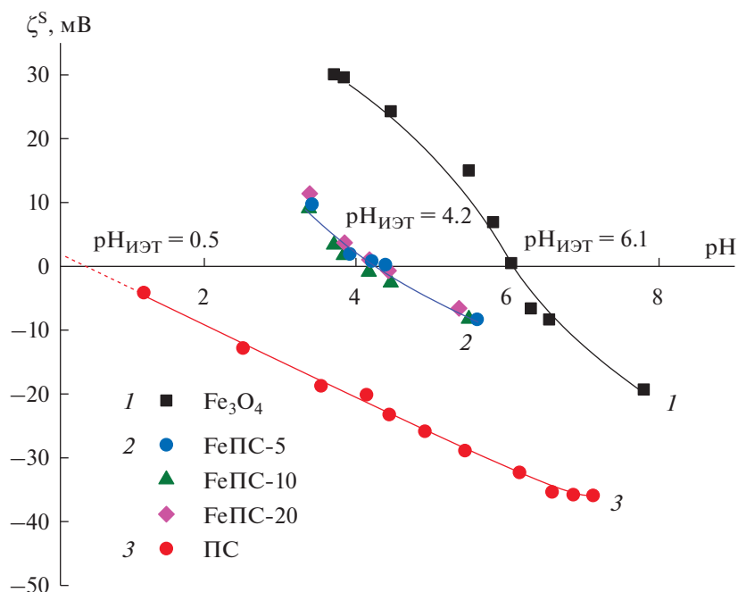
Рис. 8. Зависимость электрокинетического потенциала \zeta^S частиц всех исследованных образцов от pH на фоне 10^{-2} М раствора NaCl.
