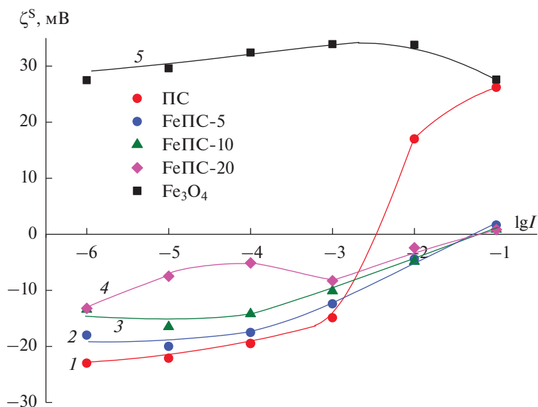
Рис. 10. Зависимость электрокинетического потенциала частиц исследованных образцов от ионной силы растворов хлорида никеля при естественном значении рН.
