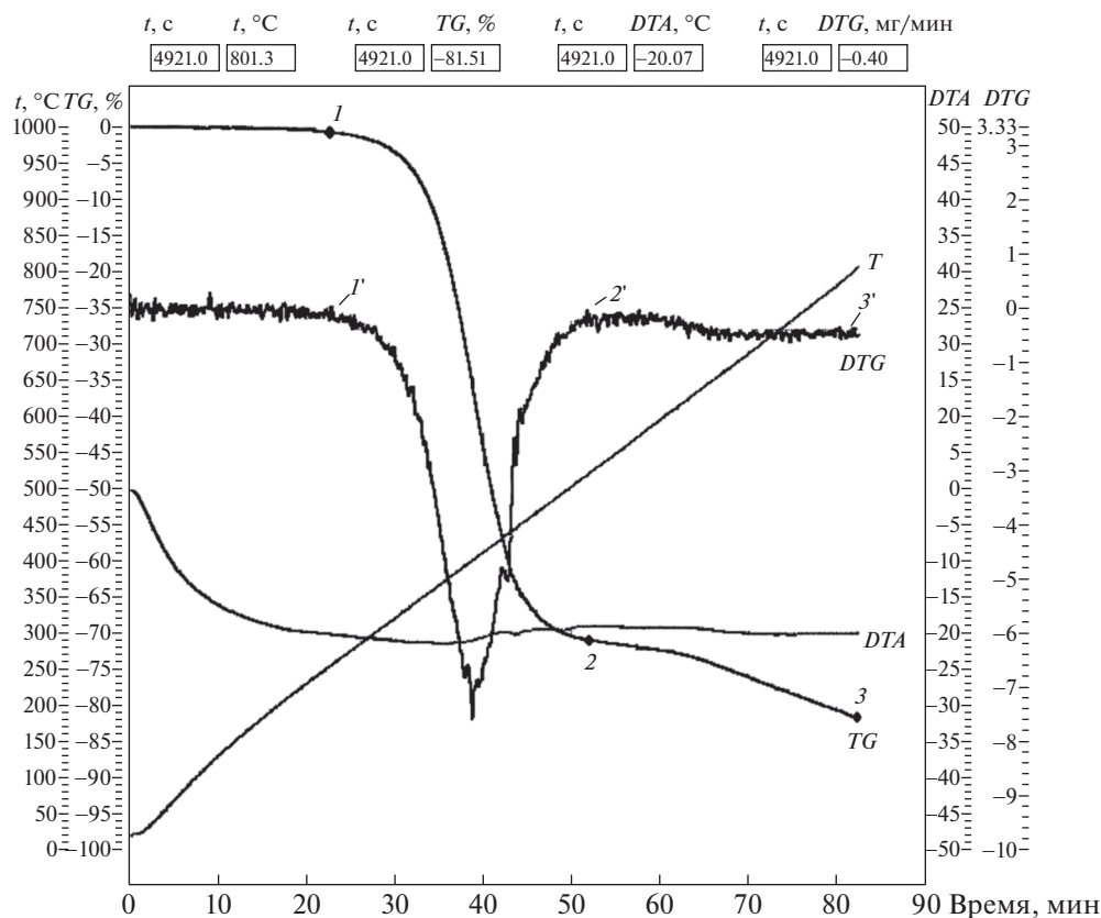
Рис. 1. Дериватограмма сланцевого пека. Потеря массы, мас. %: 1 – 0,7, 2 – 70,9, 3 – 81,4; температура, °C: 1' – 255, 2' – 520, 3' – 800.
