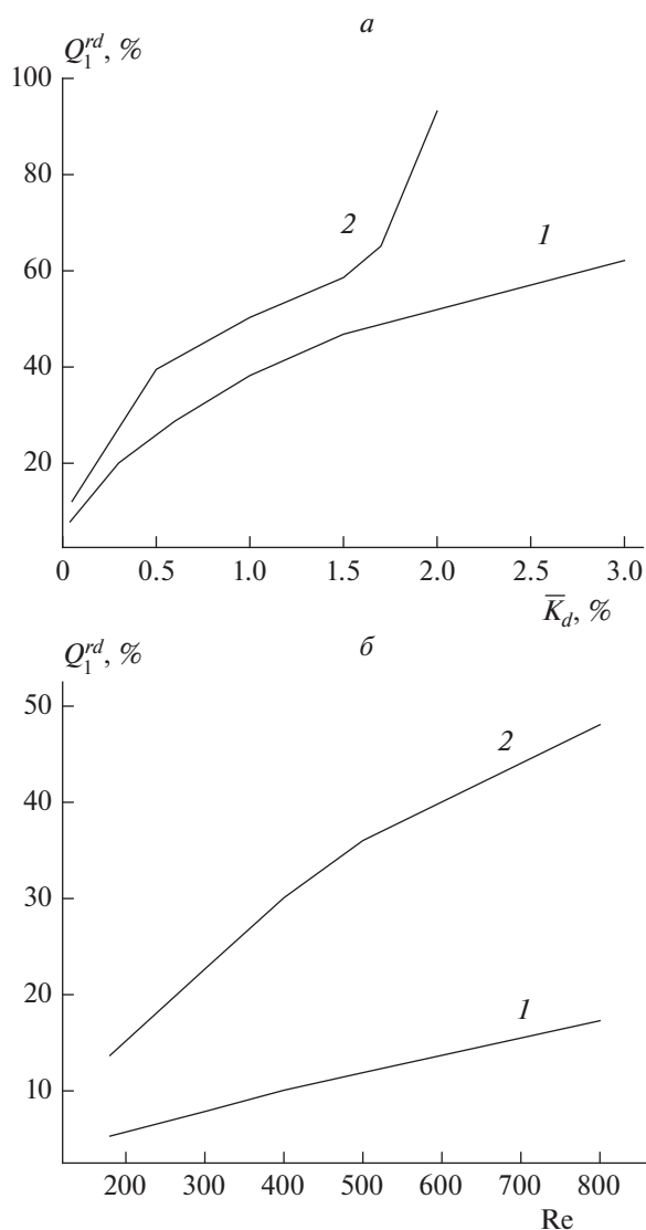
Рис. 2. Поведение коэффициента хаотичности Q_1^{rd} : а – зависимость Q_1^{rd} от \bar{K}_d , кривая 1 рассчитана при Re = 300 , кривая 2 – при Re = 500 ; б – зависимость Q_1^{rd} от Re , кривая 1 рассчитана при \bar{K}_d = 0.04\% , кривая 2 – при \bar{K}_d = 0.4\% .
