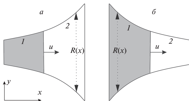
Рис. 1. Схема горения слоев: u — скорость фронта, 1 — продукты горения, 2 — непрореагировавшая смесь, стрелки — направление распространения горения; а — зона реакции растягивается, б — сжимается.
