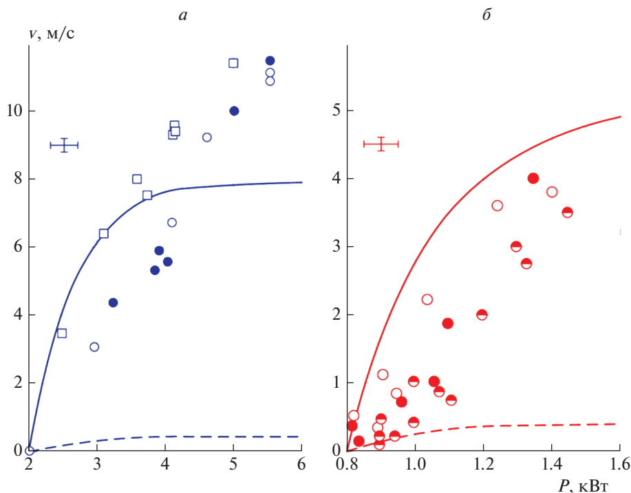
Рис. 1. Сравнение экспериментально наблюдаемых предельных скоростей распространения волн светового горения, v , при заданной мощности лазерного излучения P с рассчитанными, u_t(P) , (штриховая линия) в модели теплопроводностного распространения и с учетом поправочного множителя u_t(P)(\rho_0/\rho_k)^{1/2} (сплошная линия) в случаях: a – воздух, 1 бар [8] и б – Ar, 1 бар [18]. Различная форма точек соответствует разным условиям фокусировки, не оказывающим существенного влияния на скорость распространения ВСГ.
