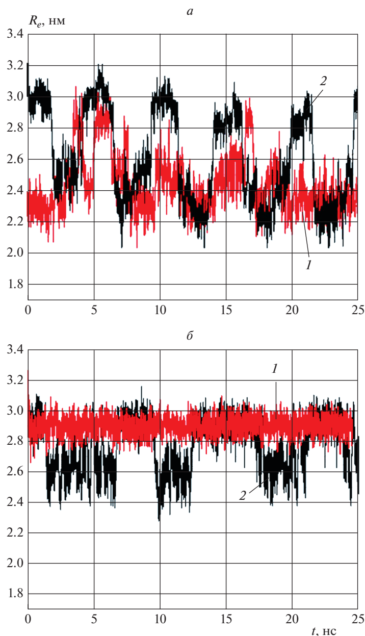
Рис. 6. Детектирование органических молекул в режиме стохастического резонанса олиго-NIPMA-30: a – динамика спонтанных вибраций (траектория 1) и стохастического резонанса (траектория 2) ненагруженного олиго-NIPMA-30; б – динамика олиго-NIPMA-30, нагруженного молекулой триптофана (номера траекторий соответствуют случаю a ).
