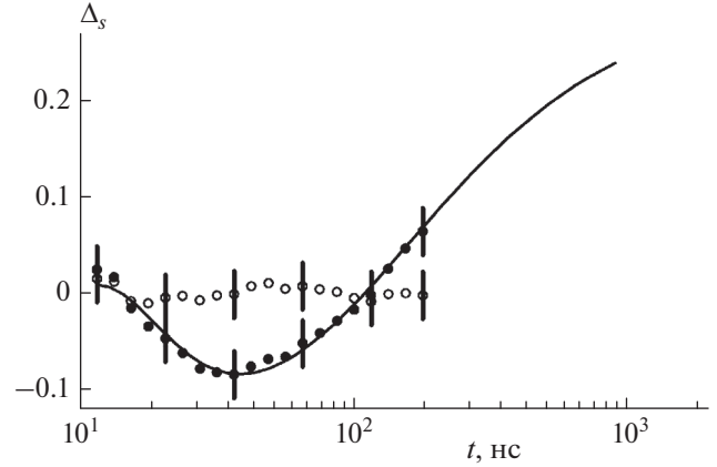
Рис. 2. Относительные отклонения \Delta_s(t) = \Delta_s^v(t) теоретических КСФ p_s^v(t) , v = c, d , от экспериментальной КСФ p_s^{exp}(t) (см. (22)), рассчитанные с использованием результатов, представленных на рис. 1. Отклонения \Delta_s^c(t) и \Delta_s^d(t) изображены светлыми и черными кружками соответственно. На графиках функций \Delta_s^c(t) и \Delta_s^d(t) короткие вертикальные линии обозначают ошибку рассчитанных отклонений (обусловленных ошибкой измерения p_s^{exp}(t) [11]). Сплошная линия — поведение относительного отклонения \Delta_s(t) = \Delta_s^{dc}(t) = p_s^d(t)/p_s^c(t) - 1 теоретических КСФ p_s^c(t) и p_s^d(t) в диапазоне времен 30 \leq t < 10^3 нс (см. разд. 3).
