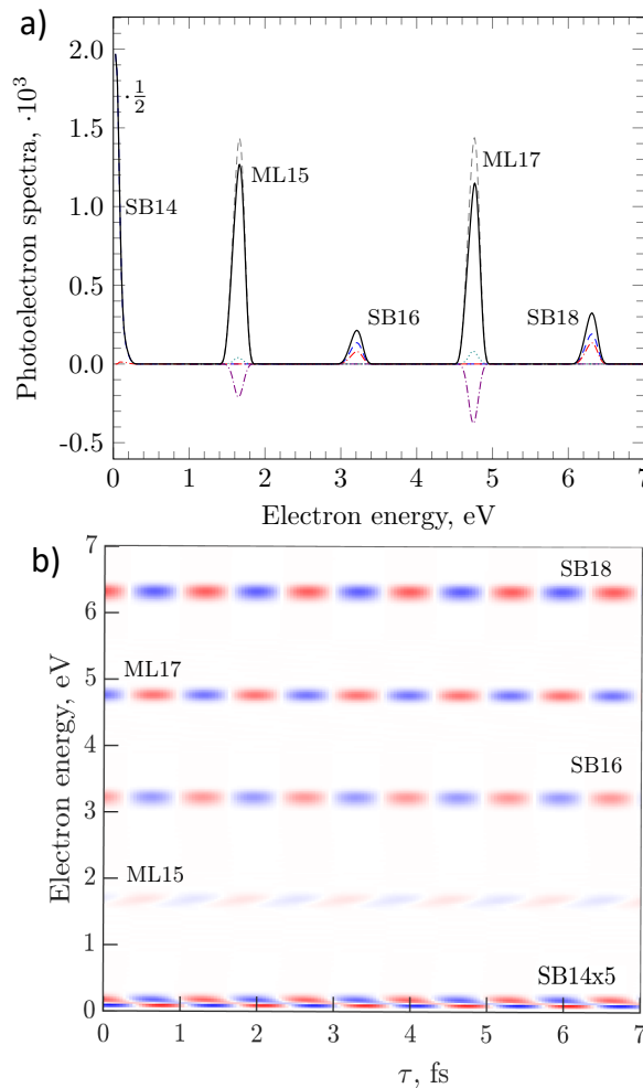
Рис. 5. a) Усредненный по фазе ИК-поля спектр при 800 нм и E_{ir} = 5 \cdot 10^{-3} ат. ед., полученный по теории возмущений. Жирная черная линия обозначает итоговый спектр; серая штриховая — первый порядок ТВ; красная штрихпунктирная — второй порядок ТВ, происходящий с испусканием ИК-фотона; синяя штриховая — второй порядок ТВ с поглощением ИК-фотона; сиреневая штрихпунктирная — вклад интерференции первого и третьего порядков; голубыми точками отмечен вклад от третьего порядка ТВ. b) Осцилляции (RABBIT traces) как функции задержки ИК-импульса и энергии фотоэлектронов. Величина осцилляций в SB14 представлена с фактором 5
