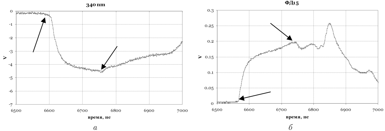
Рис. 2. Осциллограммы свечения фронта ударной волны в азотном флюиде в эксперименте при давлении 230 ГПа: a — сигнал фотоумножителя на длине волны 340 нм; б — сигнал фотодиода
