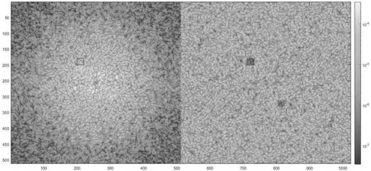
Рис. 3. Результаты моделирования (тривиальной зональной) коррекции волнового фронта, содержащего спекл-поле. Слева — некорректированное спекл-поле в плоскости изображения после интерференционного коронографа, где красным квадратом показана область коррекции. Справа — ослабленное спекл-поле в зоне коррекции и симметричной области для интерференционного коронографа по схеме интерферометра вращательного сдвига (ИВС 180°), см. [2]
