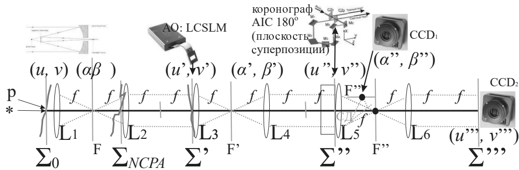
Рис. 5. Принципиальная оптическая схема коррекции ВФ, содержащая телескоп, корректор ВФ (АО), интерференционный коронограф, CCD-камеры для регистрации изображений в фокусе и в зрачке
