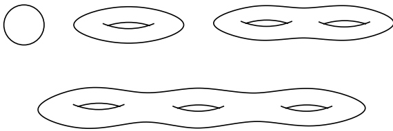
Рис. 2. Абстрактные поверхности рода 0, 1, 2, 3
