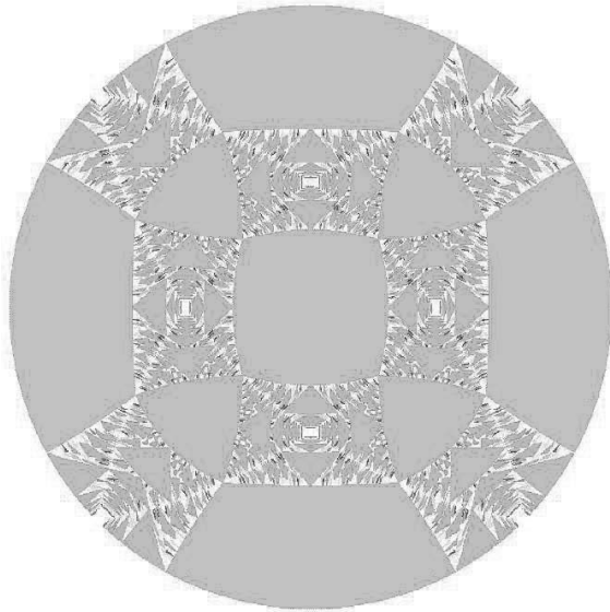
Рис. 15. Угловая диаграмма для поверхности \cos p_x + \cos p_y + \cos p_z = 0 [44]
