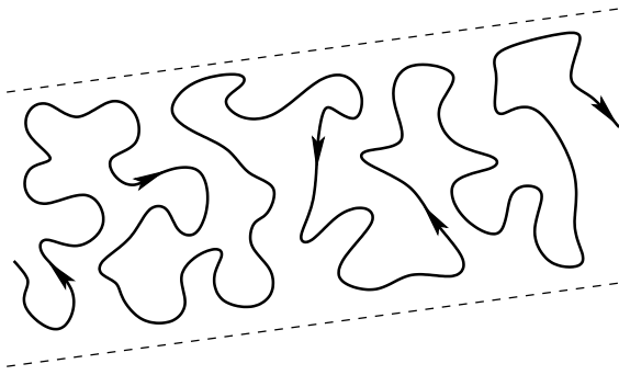
Рис. 5. Устойчивая открытая траектория в плоскости, ортогональной \mathbf{V} (схематично)
