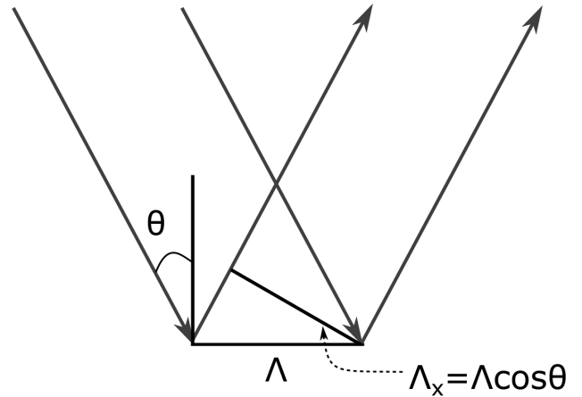
Рис. 3. К геометрии размера пучка, отраженного от SLM
