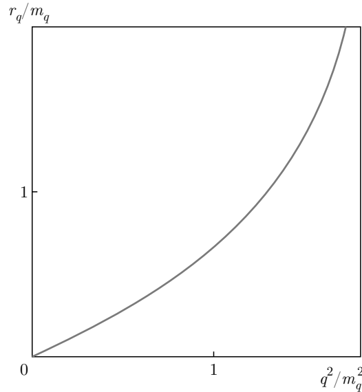
Рис. 1. Зависимость радиуса заряженной сферы r_q от q^2 в единицах массы m_q , см. (22)
