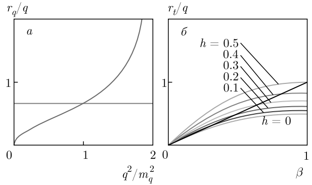
Рис. 2. а) Зависимость r_q/q от q^2/m_q^2 . б) Зависимости r_t/q от \beta при разных h для неравенства (59)
