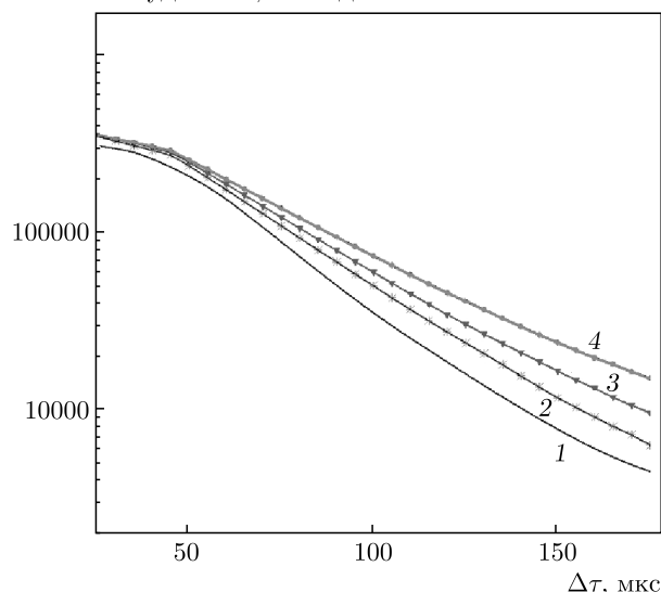
Рис. 7. Огибающие спинового эха (в логарифмическом масштабе) для линии перехода \nu_1 (2) в спектре ЯКР ^{209}\text{Bi} соединения \text{Bi}_2\text{S}_3 (табл. 2) во внешних магнитных полях H_{ext} : 1 — H_{ext} = 0 , 2 — H_{ext} = 10 Э, 3 — H_{ext} = 15 Э, 4 — H_{ext} = 40 Э
