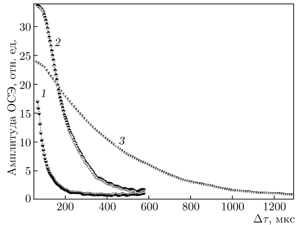
Рис. 1. Огибающие спинового эха для линии ЯКР ^{209}\text{Bi} перехода \nu_2 ( \Delta m = 3/2-5/2 ) в спектре чистого монокристалла BGO в нулевом поле (1) и H_{ext} = 30 Э (2), а также в BGO, легированном празеодимом, в нулевом поле (3) [38]
