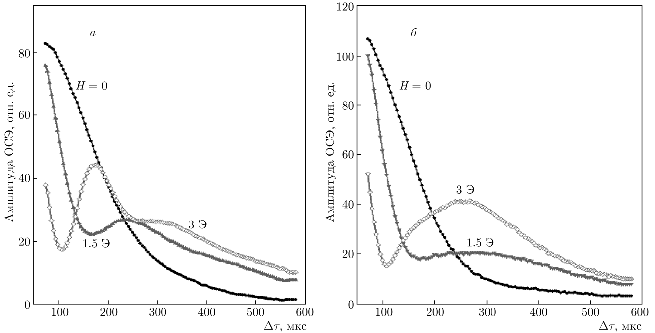
Рис. 4. Огибающие спинового эха для линий переходов \nu_1 (1) (а) и \nu_1 (2) (б) в спектре ЯКР ^{121}\text{Sb} соединения \text{Sb}_2\text{S}_3 (табл. 2) во внешних магнитных полях указанных напряженностей [28]
