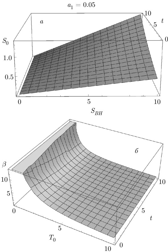
Рис. 1. Соотношения между S_0 , S_{BH} и t (а) и между \beta , T_0 и t (б) при a_1 = 0.05
