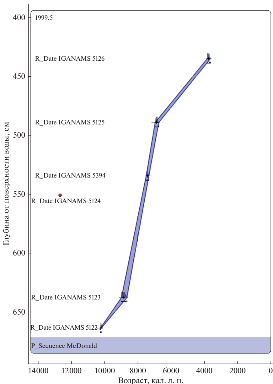
Рис. 3. Глубинно-возрастная модель донных отложений оз. Конюховского (OxCal v 4.4.4.). Красной точкой отмечена инверсия дат.
