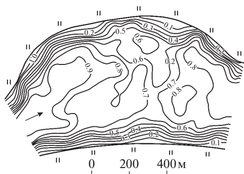
Рис. 4. Структура потока в привершинной части синусоидальной Войкарской излучины.
