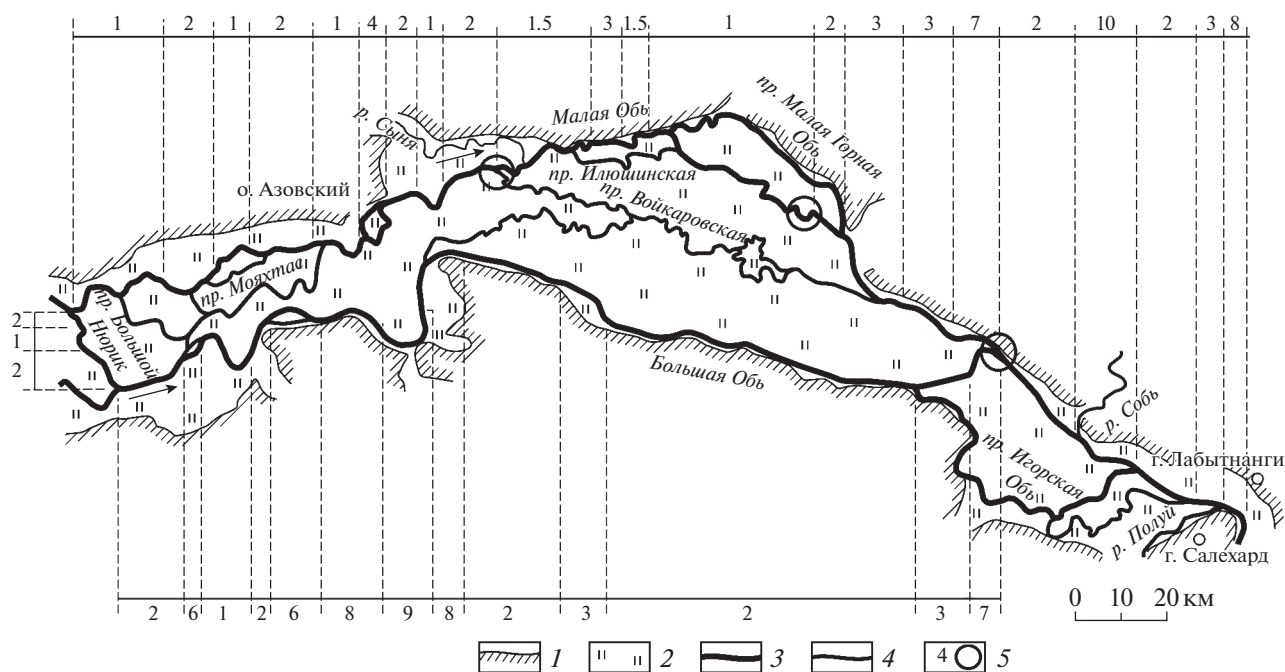
Рис. 1. Общая схема. 1 – коренные берега; 2 – пойма; 3 – рукава развоенного русла; 4 – пойменные протоки и притоки; 5 – положение участков русла на рис. 4, 6, 7; морфодинамические типы рукавов развоенного русла нижней Оби: 1 – прямолинейное неразветвленное русло; излучины: 2 – свободные, 3 – вписанные, 4 – вынужденные, 5 – обтекающие; русловые разветвления: 6 – одиночные, 7 – параллельно-рукавные, 8 – “дельтовые”, 9 – односторонние, 10 – пойменно-русловые.
