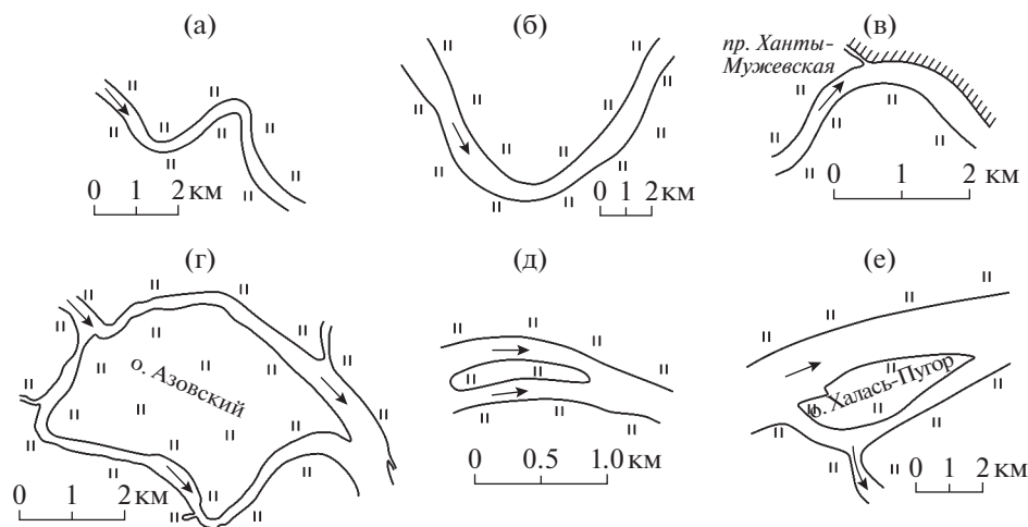
Рис. 2. Морфодинамические типы русла Малой Оби. Излучины: а) сегментная, б) синусоидальная, в) вынужденная; разветвления: г) пойменно-русловое, д) одиночное, е) одностороннее.
