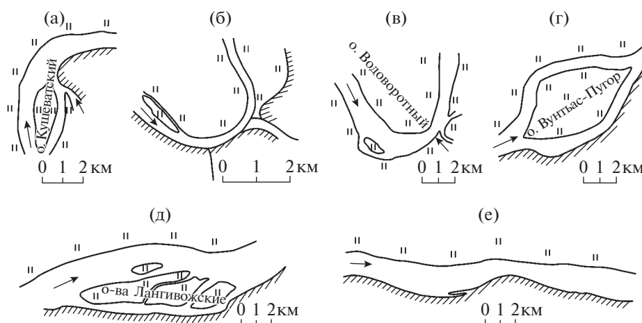
Рис. 3. Морфодинамические типа русла Большой Оби. Излучины: а) обтекающая, б) вписанная, в) свободная; разветвления: г) одиночное, д) одностороннее; е) прямолинейное неразветвленное.
