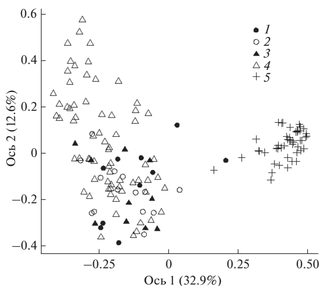
Рис. 3. Ординация проб в пространстве первой и второй главной координат (в скобках приведена доля объясняемой дисперсии). Участки и микростации: 1 – внутри стволов, 2 – почва под стволами, 3 – почва рядом со стволами, 4 – почва на постоянных пробных площадях на территории “люмбрицидной пустыни”, 5 – почва на фоновой территории.
