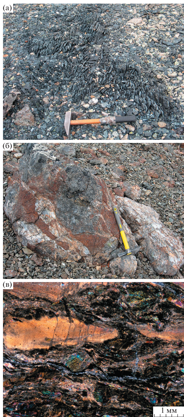
Рис. 2. Породы приконтактной тектонизированной зоны массива.
