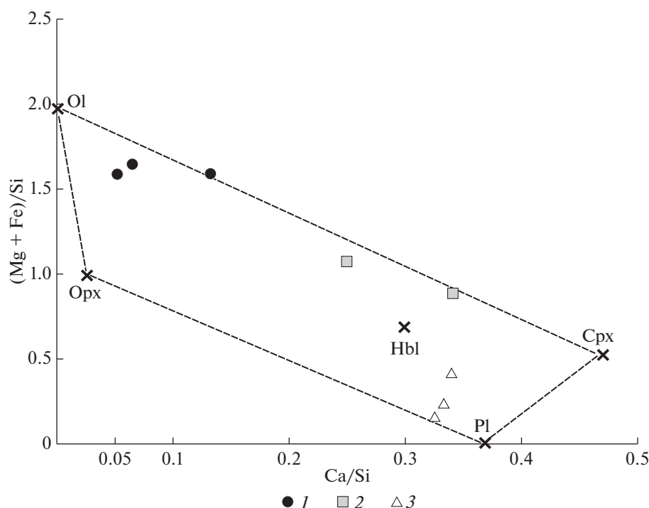
Рис. 9. Диаграмма Ca/Si—(Mg + Fe)/Si для валовых составов пород и первичных минералов из пород массива руч. Луковский.
