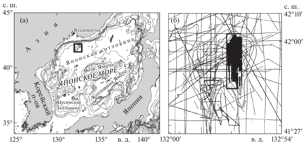
Рис. 1. Местоположение района работ (а) в Японском море (показано прямоугольником, батиметрия GEBCO [1]) и расположение профилей эхолотного промера (б) в районе возвышенности Первенец, полученных с помощью судовых однолучевых эхолотов (показаны тонкими линиями) и полигона работ (обозначен прямоугольником) с многолучевым эхолотом SeaBeam 3050 (батиметрия из [2]).
