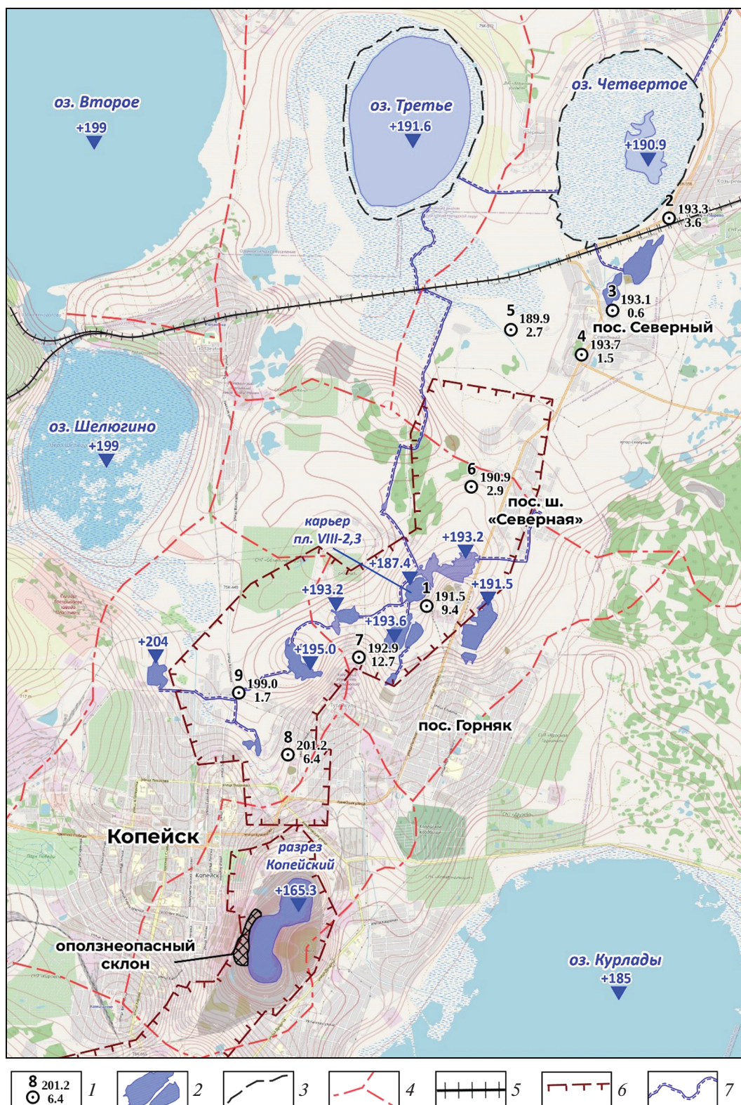
Рис. 2. Ситуационная схема и размещение техногенных объектов в районе ш. «Красная горнячка». 1 – наблюдательная скважина: вверху номер, справа: вверху абс. отм. уровня воды, внизу глубина до воды; 2 – затопленные карьеры и провалы; 3 – контур озер на 2003 г.; 4 – границы частных водосборов; 5 – железная дорога; 6 – граница горного отвода; 7 – дренажные канавы.
