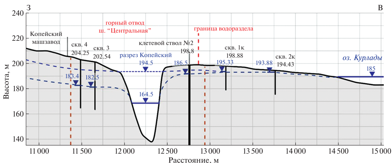
Рис. 7. Схематический разрез по линии Копейский машзавод – разрез Копейский – оз. Курлады.
