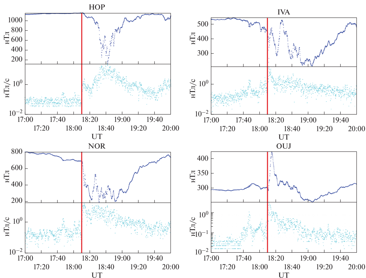
Рис. 2. Минутные магнитограммы X -компоненты (верхние графики) для выбранных станций (HOP, NOR, IVA, OUI) сети IMAGE. Вариабельность магнитного поля dH/dt (нижние графики) для этих же станций. Начало интервала 1700 UT, конец интервала 2000 UT. Начало взрывной фазы суббури отмечено красной вертикальной линией.
