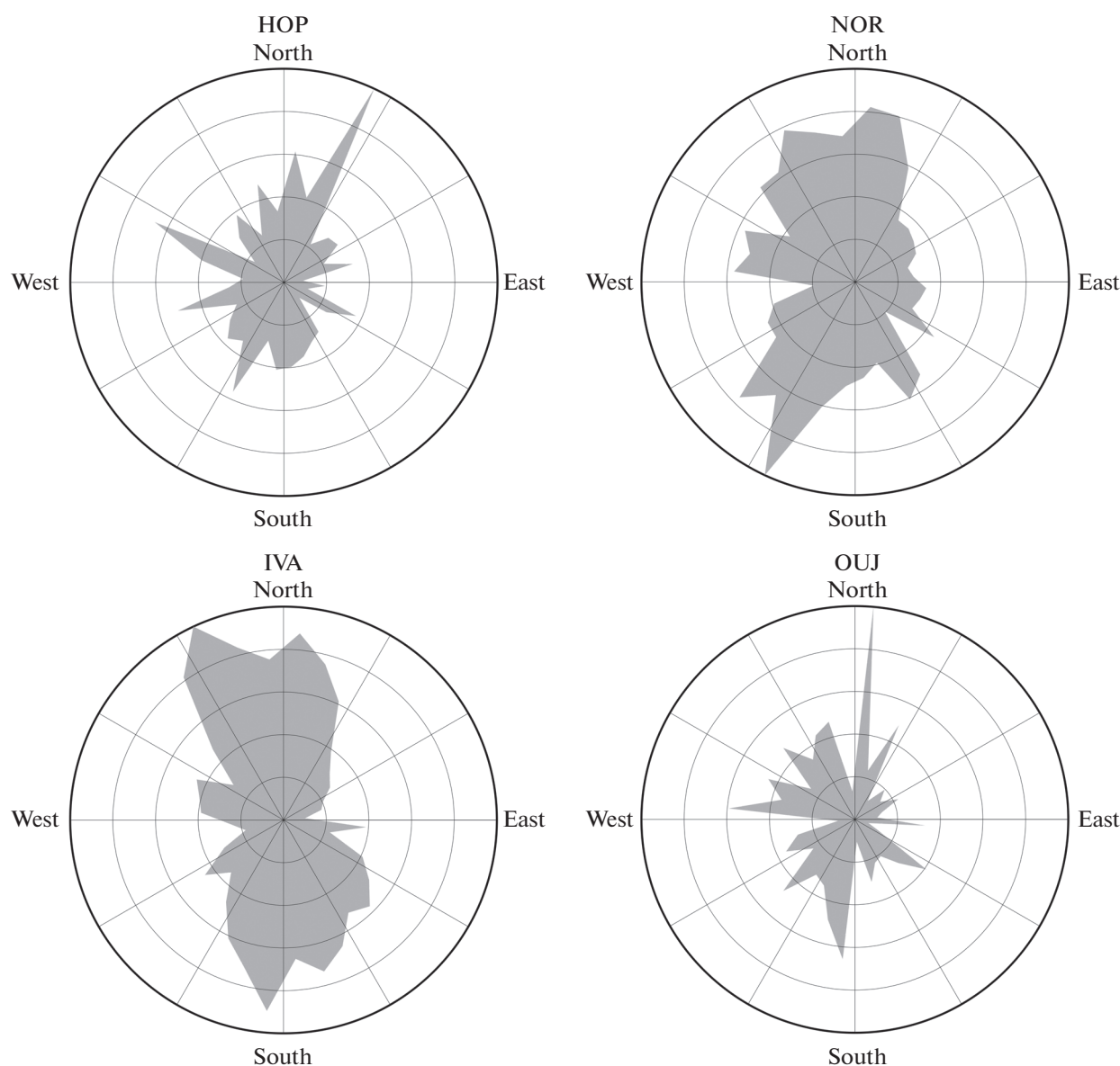
Рис. 4. Полярные 2D-диаграммы горизонтальных компонент d\mathbf{B}_t/dt на поверхности Земли (плоскость XY , окружность единичного радиуса) для станций HOP, NOR, IVA, OUI на взрывной фазе суббури (интервал 1810–2000 UT). Ориентация осей соответствует ориентации исходных геомагнитных данных.
