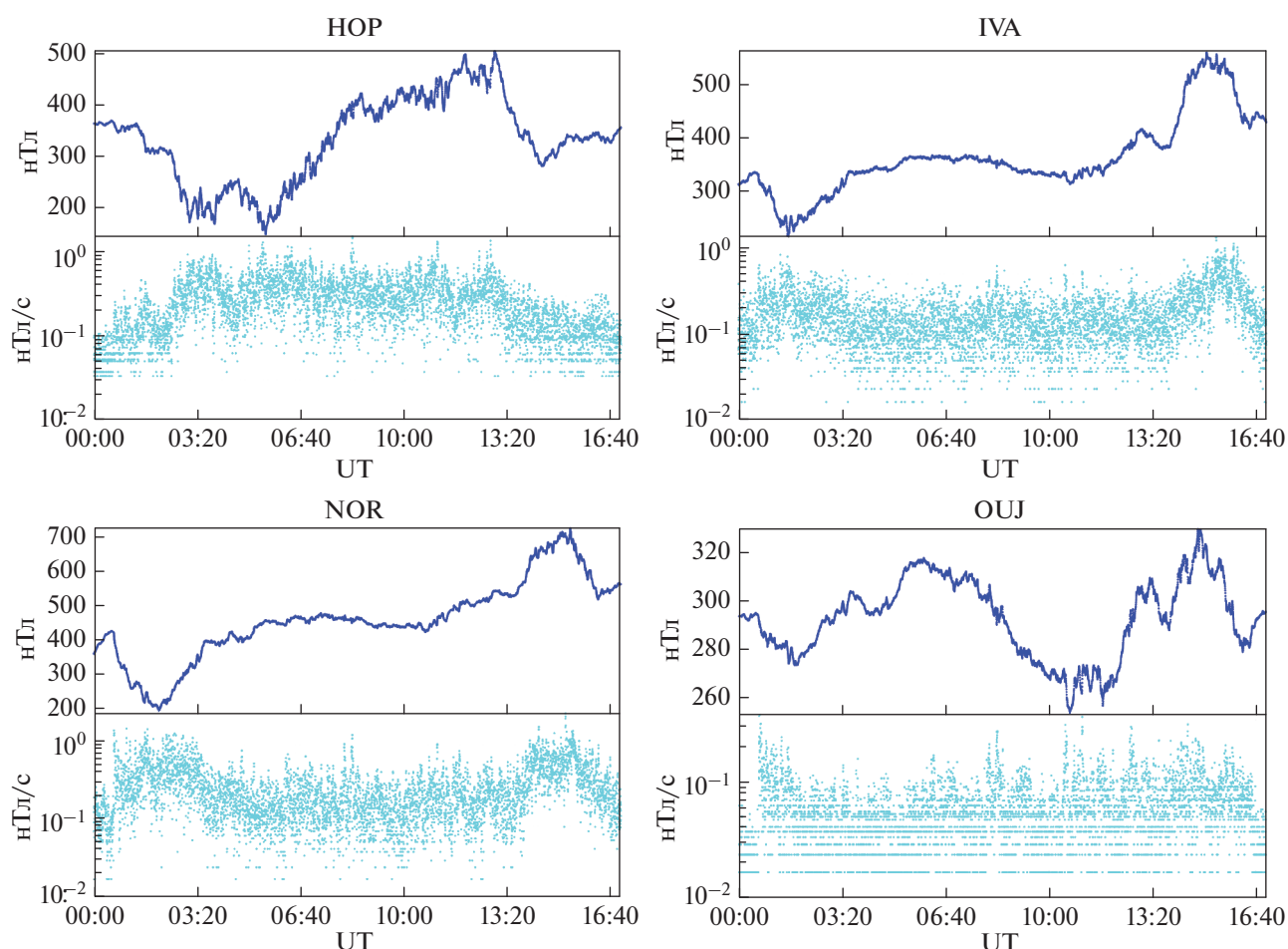
Рис. 1. Минутные магнитограммы X -компоненты (верхние графики) для выбранных станций (HOP, NOR, IVA, OUI) сети IMAGE. Вариативность магнитного поля dX/dt (нижние графики) для этих же станций. Начало интервала 0000 UT, конец интервала 1700 UT.
