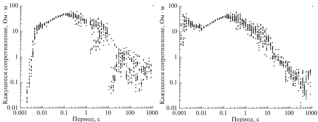
Рис. 7. Сравнение двух результатов обработки данных МТЗ в точке № 15 профиля Тихвин–Винницы по программе EPI-KIT [Епишкин, 2018] на примере оценок эффективной компоненты кажущегося сопротивления: (а) — одиночная обработка; (б) — обработка с использованием синхронных записей электрического и магнитного поля в базовой точке п. Алеховщина (рис. 2).
