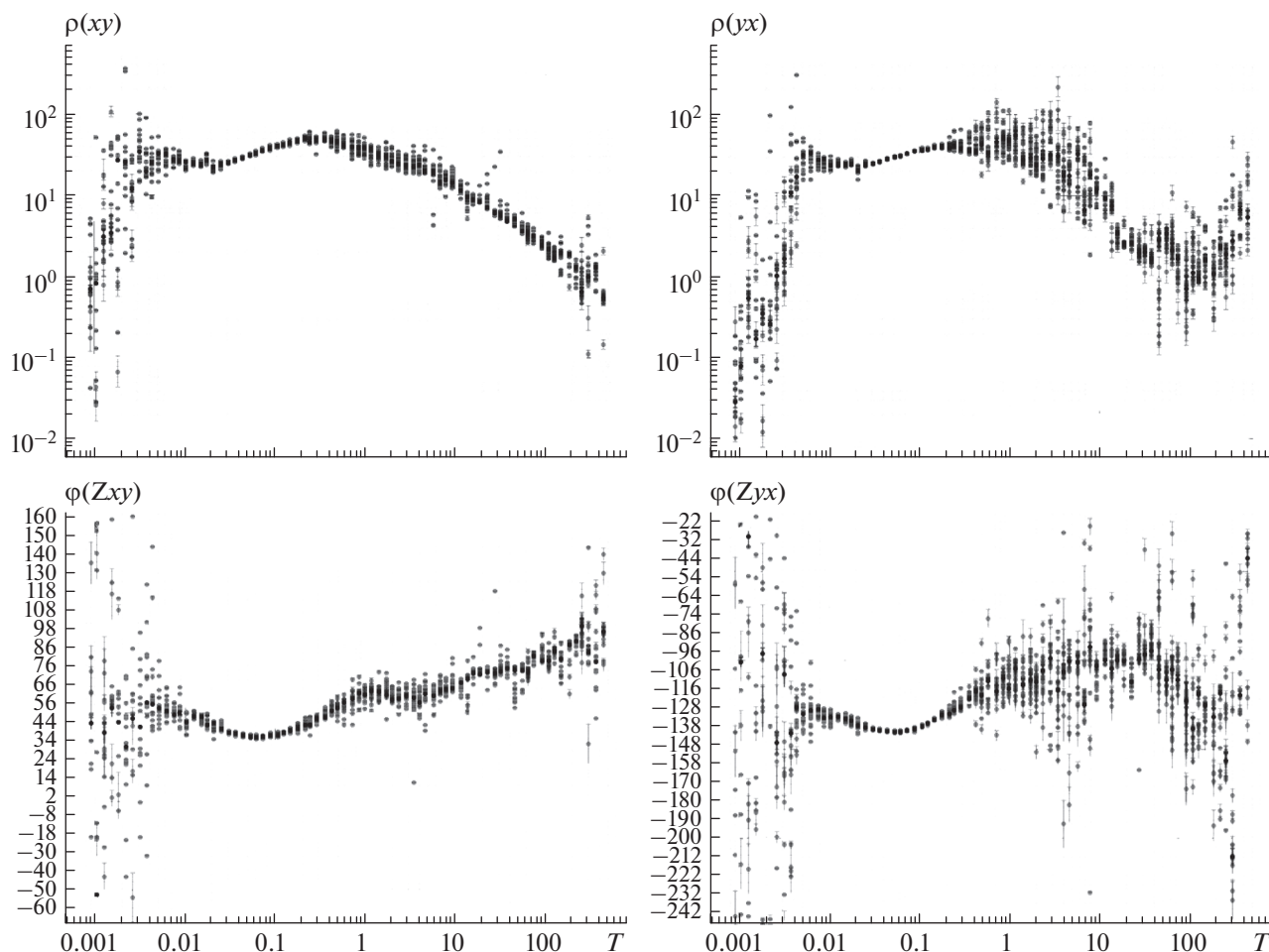
Рис. 4. Пример обработки данных в программе ERI-KIT: облака оценок фаз главных компонент импеданса и соответствующих кажущихся сопротивлений, полученных по множеству последовательных равных интервалов временного ряда, с доверительными интервалами. Черным цветом показаны средние значения. Направления X и Y соответствуют измерительным осям.
