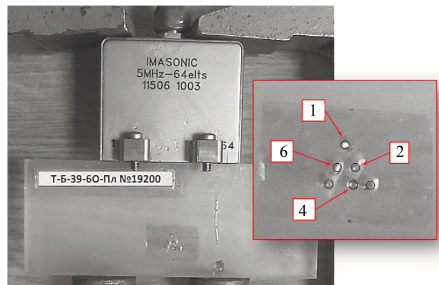
Рис. 5. Фотография образца и используемой АР.
