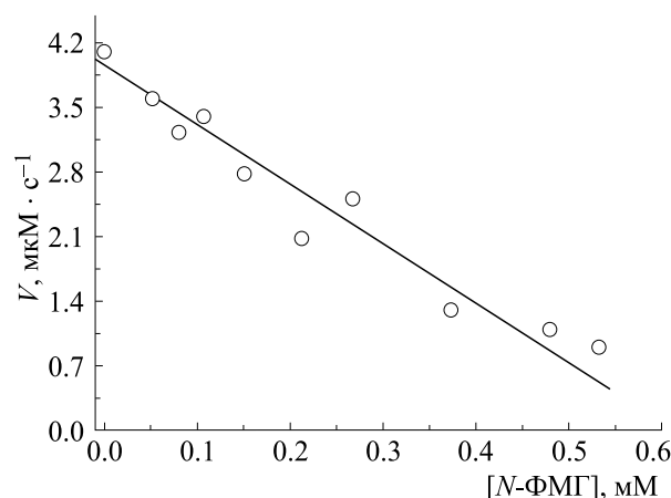
Рис. 4. Зависимость скорости окисления гидрохинона ( 0.05 \div 0.4 мМ) на ферменте ПХ (15 нМ) в присутствии 0.64 мМ \text{H}_2\text{O}_2 от концентрации ингибитора N -ФМГ ( 0.05 \div 0.53 мМ). Среда — 0.05 М Na-ацетатный буфер, pH 5.4.
