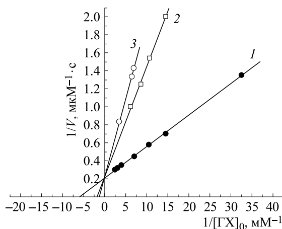
Рис. 5. Зависимость обратной скорости ферментативной реакции от обратной концентрации ингибитора N -ФМГ (координаты Лайнуивера—Берка): 1 — без ингибитора, 2 — в присутствии 0.31 мМ N -ФМГ, 3 — в присутствии 0.398 мМ N -ФМГ. Концентрации реагентов: ПХ — 20 нМ, \text{H}_2\text{O}_2 — 0.62 мМ, гидрохинон — 0.07 \div 0.285 мМ, среда — 0.05 М Na-ацетатный буфер, pH 5.4.
