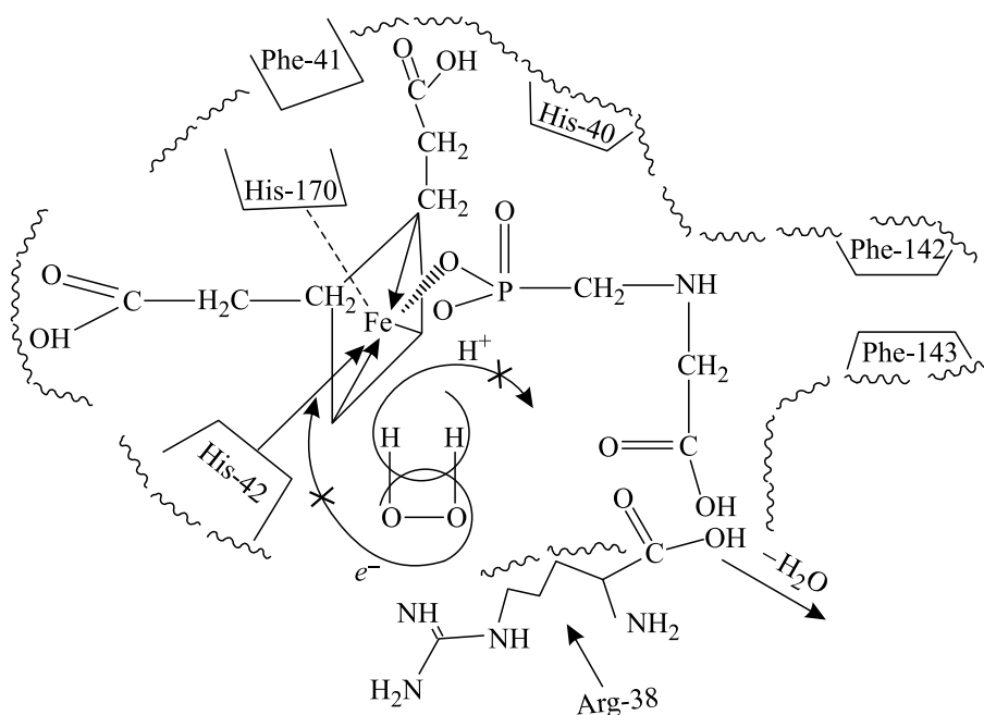
Рис. 6. Гипотетическая схема ингибирования активности ПХ N-ФМГ.
