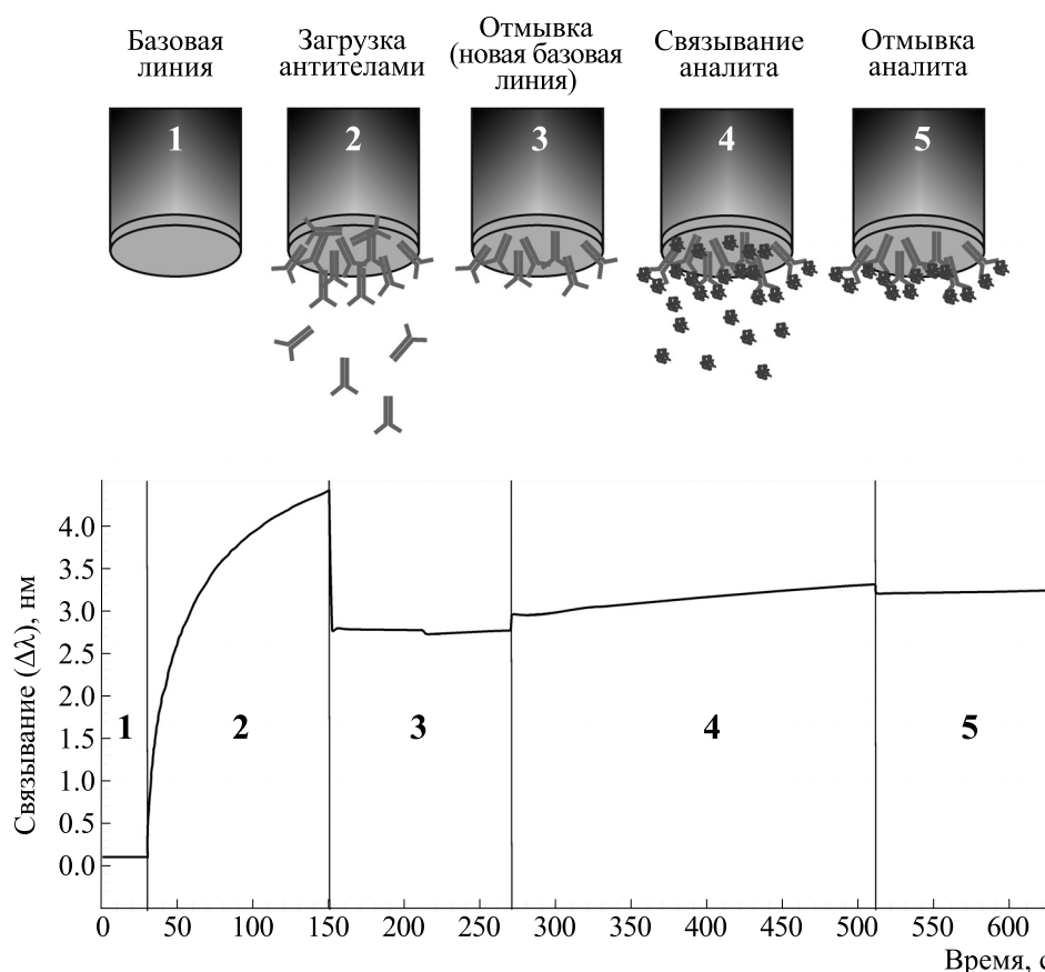
Рис. 2. Схема протокола определения концентрации растворенного фактора роста VEGF-A методом BLI. Протокол включает пять этапов: 1 – регистрация начальной базовой линии (в PBS); 2 – загрузка биосенсора с протеином А антителами против VEGF-A (стоковый раствор антител); 3 – отмывка биосенсора от слабо связавшихся антител и определение новой базовой линии (сначала в PBS, затем – в среде с сывороткой); 4 – детекция VEGF-A в образце (в кондиционированной среде с сывороткой); 5 – отмывка от VEGF-A (в среде с сывороткой).
