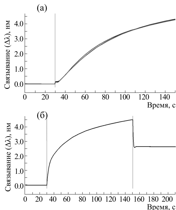
Рис. 3. Первичная загрузка биосенсоров с протеином А антителами против VEGF-A мыши. Профили связывания четырех биосенсоров с антителами (а) и вид типичной кривой связывания-диссоциации (б).
