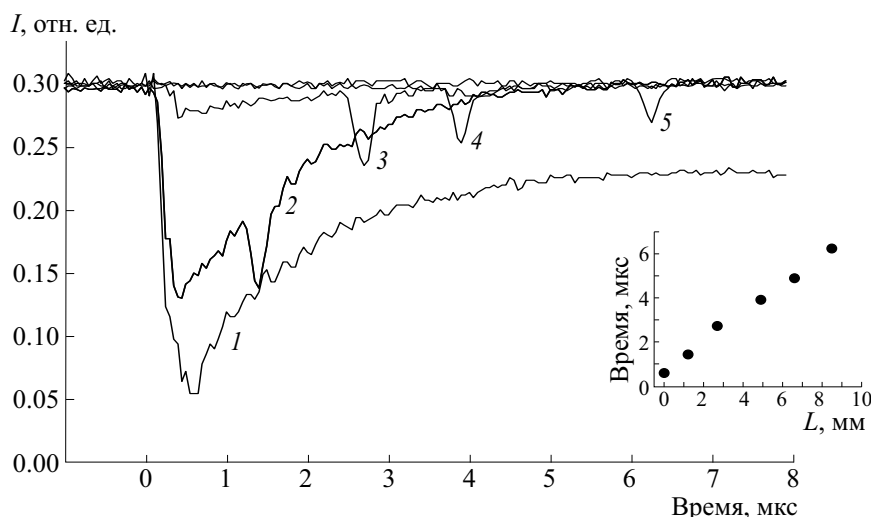
Рис. 2. Временные зависимости интенсивности нерассеянной части зондирующего луча в физиологическом растворе с эритрозином ( C = 0.25 мМ) на разных расстояниях L от перетяжки возбуждающего пучка ( P = 20 МВт/см 2 ): 1 — L = 0 мм; 2 — L = 1.2 мм; 3 — L = 2.7 мм; 4 — L = 4.9 мм; 5 — L = 8.5 мм. На врезке — зависимость времени прихода волны от расстояния до перетяжки.
