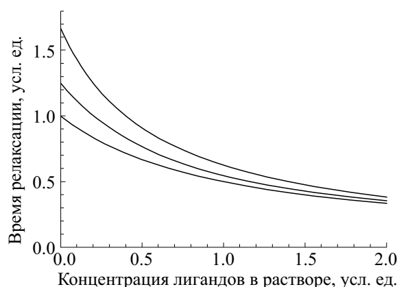
Рис. 2. Зависимости времени релаксации от концентрации лигандов в растворе. Графики рассчитаны по формуле (16) при n = 1 . Нижняя кривая соответствует детерминированному случаю, когда отсутствует внешний шум ( \sigma_c = 0 ). Средняя кривая соответствует случаю, когда C = D = 0.2 , верхняя кривая — C = D = 0.4 .
