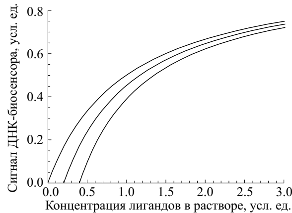
Рис. 1. Зависимости сигнала ДНК-биосенсора Y от концентрации лигандов в растворе X . Графики рассчитаны по формуле (15) при n = 1 . Верхняя кривая соответствует детерминированному случаю, когда отсутствует внешний шум ( \sigma_c = 0 ). Средняя кривая соответствует случаю, когда C = D = 0.2 , нижняя кривая когда C = D = 0.4 .
