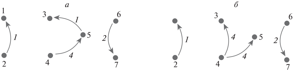
Рис. 2. Два леса — a и б , состоящие из трех исходящих деревьев с корнями 2, 4 и 6.
