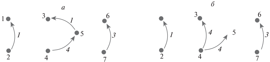
Рис. 3. Два леса — a и б , состоящие из трех исходящих деревьев с корнями 2, 4 и 7.
