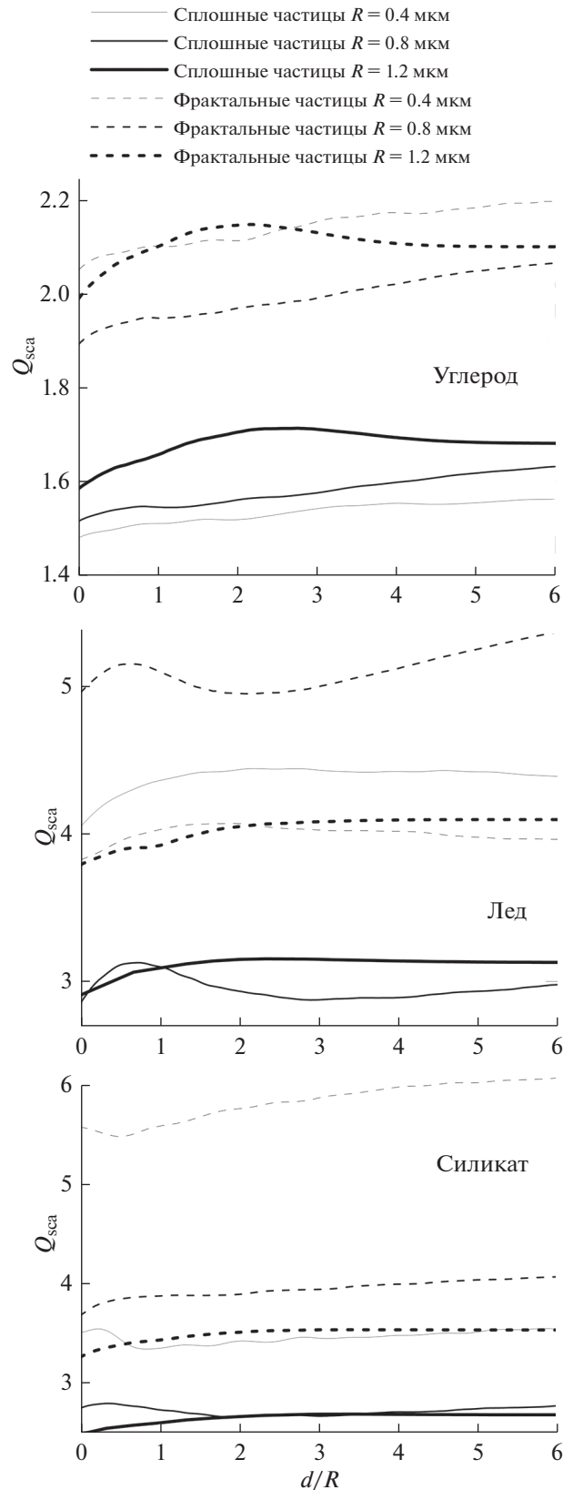
Рис. 7. Фактор рассеяния Q_{sca} как функция расстояния между частицами углерода (верхняя панель), льда (средняя панель) и силиката (нижняя панель).
