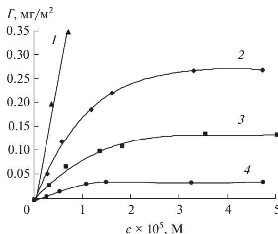
Рис. 3. Изотермы адсорбции человеческого сывороточного альбумина на кремнеземе, модифицированном: 1 — полиэтиленимином; 2 — немодифицированным; 3 — 3-аминопропилтриэтоксисиланом; 4 — метилтриэтоксисиланом [39].
