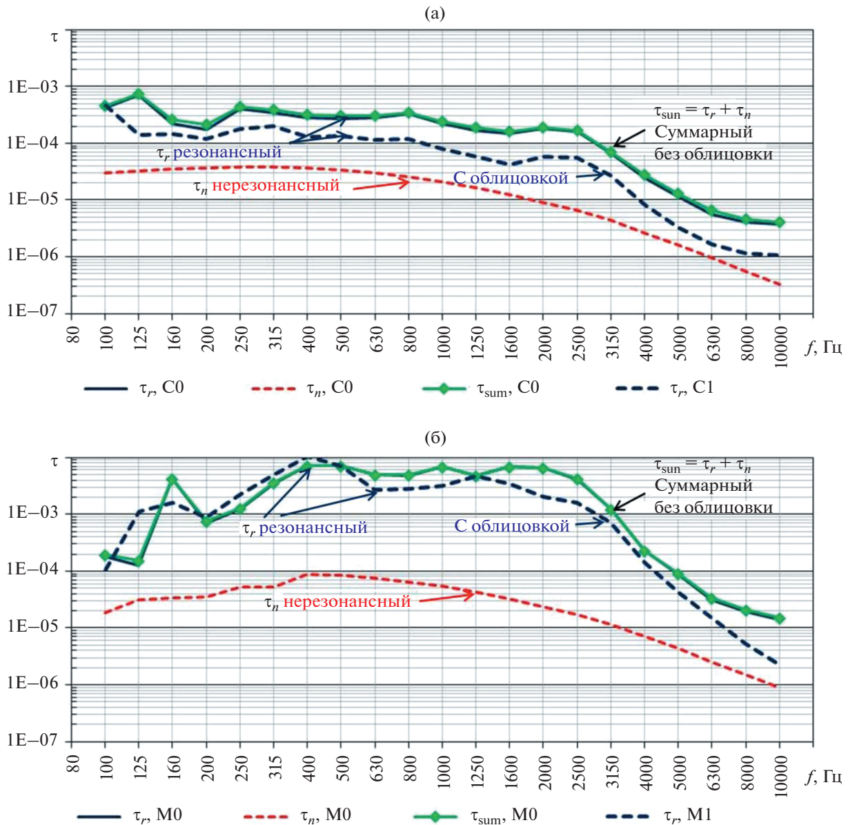
Рис. 9. Коэффициенты прохождения (а) – для композитной панели в потоке и (б) – для металлической панели в потоке.
