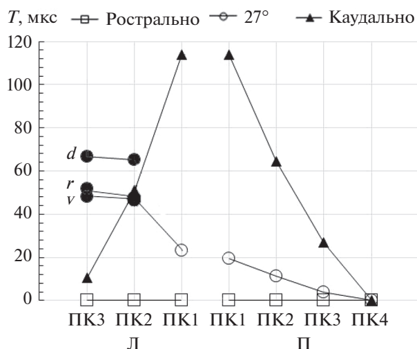
Рис. 3. Относительное время задержки парциальных звуков ПК1–ПК3 левого (Л) и ПК1–ПК4 правого (П) наружного уха, для роstralного, каудального, и под углом 27° к оси X звука во фронтальной плоскости (рис. 1), соответственно. Ось ординат – время задержки T в мкс. Ось абсцисс – номера соответствующих ПК. Маркеры, не залитые (залитые) черным, означают освещение звуком (экранирование роstrумом) соответствующих ПК. Обозначения d , r и v указаны на рис. 2.
