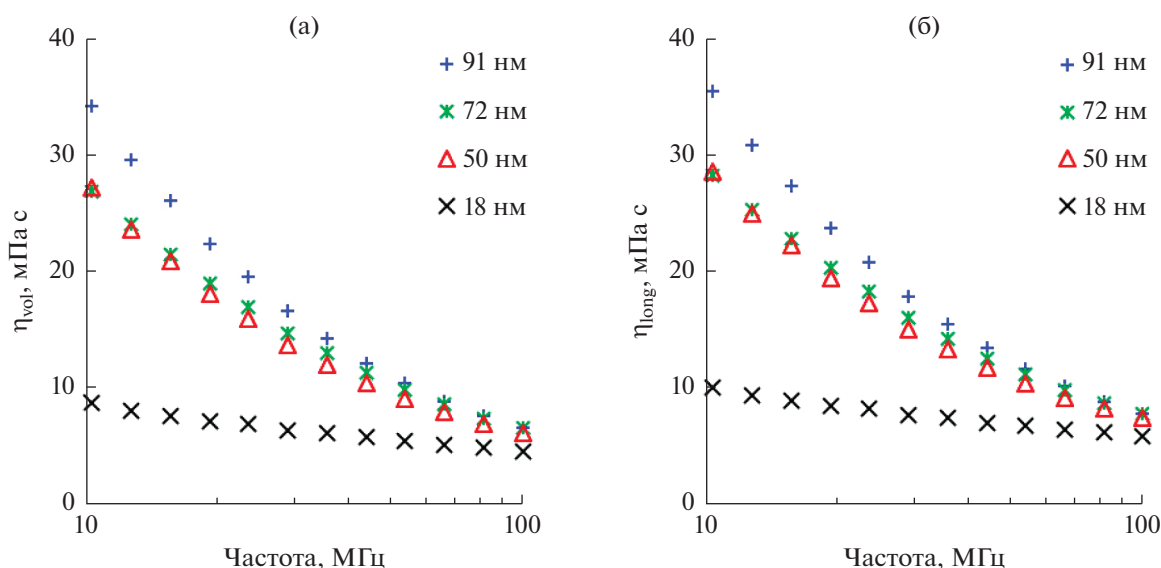
Рис. 7. Зависимость объемной вязкости наносuspензий с наночастицами (а) – \text{SiO}_2 и (б) – \text{Al}_2\text{O}_3 при их объемной концентрации 1% от частоты ультразвука.
