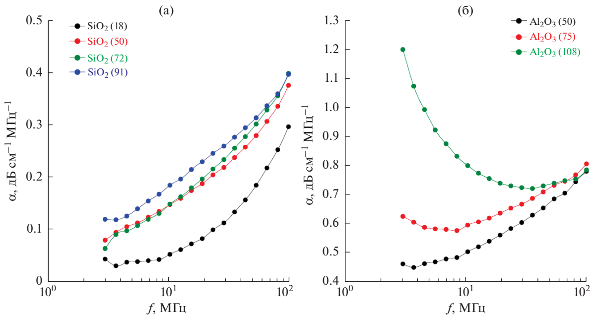
Рис. 6. Спектры коэффициента поглощения ультразвука в суспензиях с наночастицами (а) – \text{SiO}_2 и (б) – \text{Al}_2\text{O}_3 различного размера при концентрации частиц 1 мас. %.
