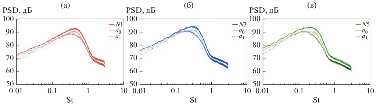
Рис. 4. Спектры ближнего поля полного сигнала (микрофоны N1 , N3 , N5 ) и его симметричной ( a_0 ) и антисимметричной ( a_1 ) составляющих для трех поперечных сечений струи: (а) – x/D = 1.5 ; (б) – x/D = 2.5 ; (в) – x/D = 3.5 . Система управления отключена.
