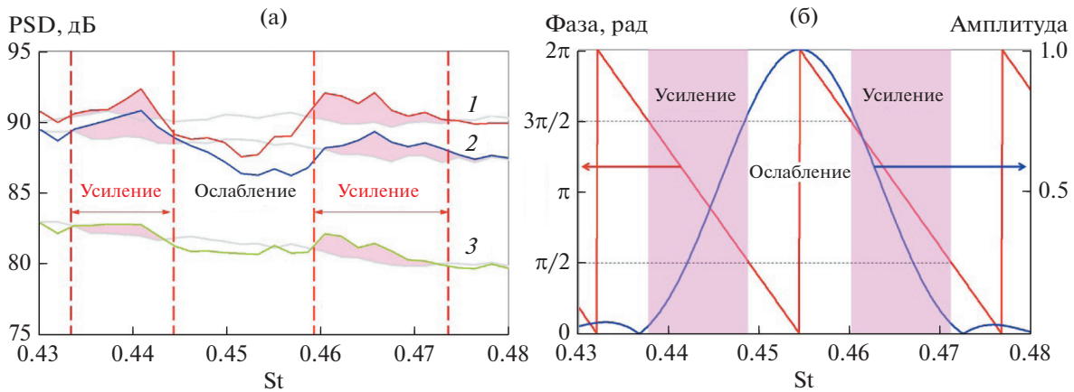
Рис. 7. Обратный эффект управления. (а) – Спектры осесимметричной моды в трех сечениях струи в режиме подавления ( 1 - x/D = 1.5 ; 2 - x/D = 2.5 ; 3 - x/D = 3.5 ). Заливкой выделены зоны усиления сигнала, серые кривые соответствуют спектрам струи без управления. (б) – Амплитудная и фазовая частотные характеристики КИХ-фильтра, заливкой выделены зоны усиления сигнала.
